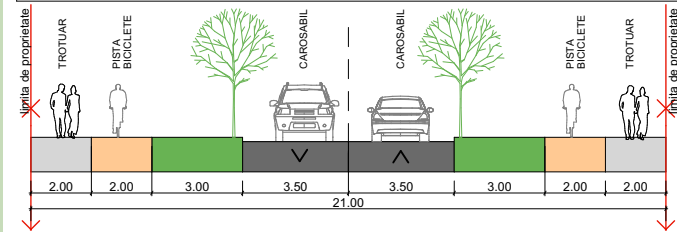
PTT 1 - Profil transversal propus prin PUZ aprobat prin HCL 323/2010 Timisoara str. Horia Hulubei - 21m
