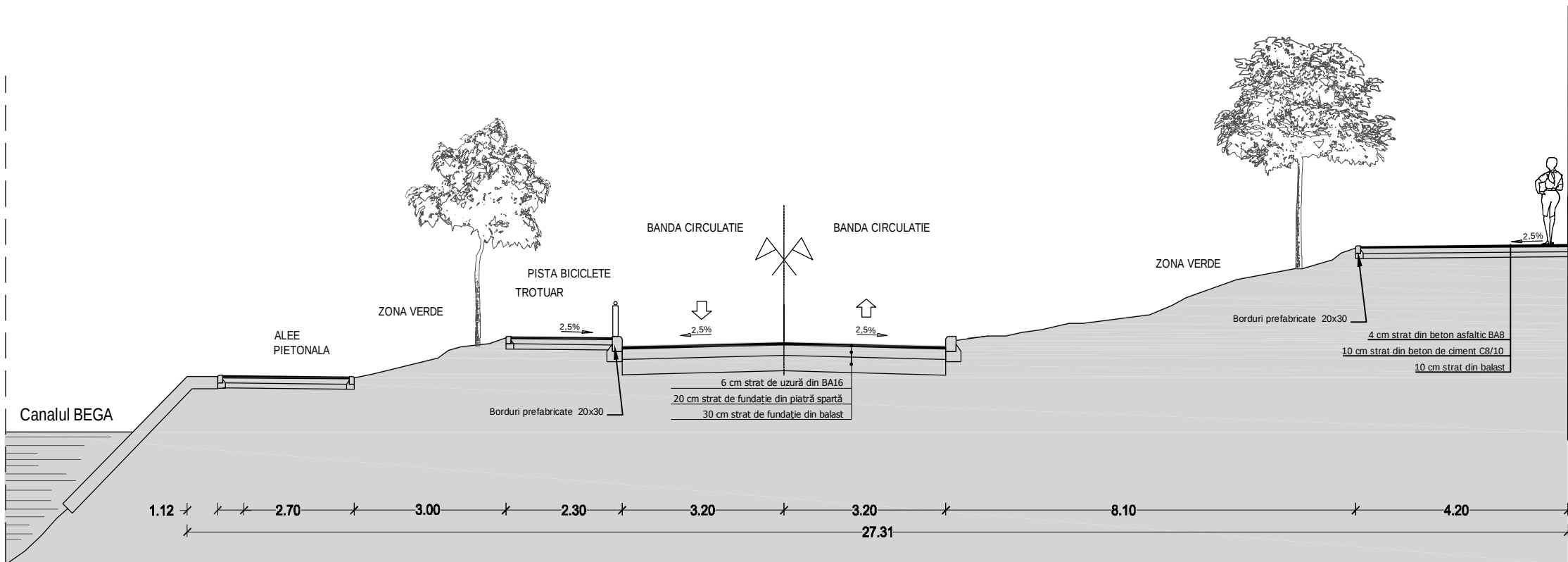
Profil Transversal 1 Splaiul Tudor Vladimirescu
