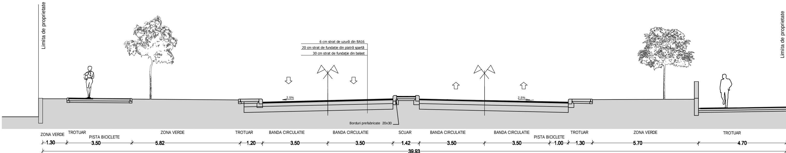
Profil Transversal Strada Iancu Văcărescu
