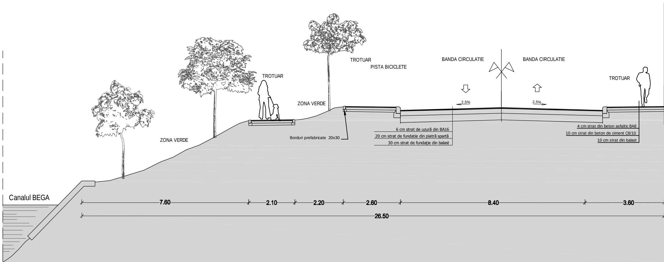
Profil Transversal 2 Splaiul Tudor Vladimirescu
