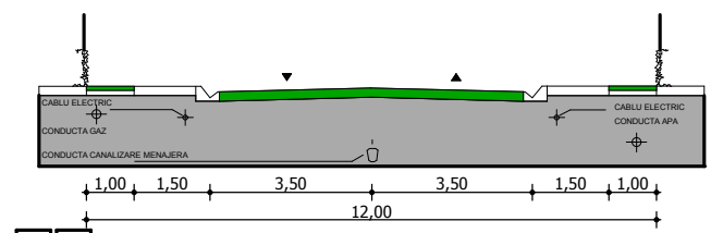
Profil transversal - strazi interioare propuse Profil drum -PUZ Locuinte Timisoara - Freidorf aprobat prin HCL 359 din 29.07.2008
