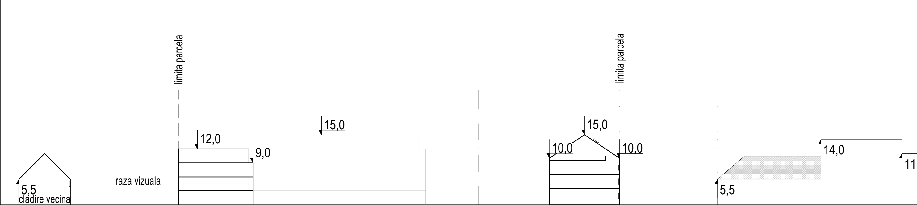
SECTIONE LONGITUDINALA AX N-S
