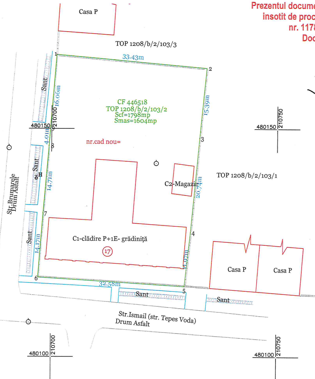
Plan de situatie Sc 1:500
