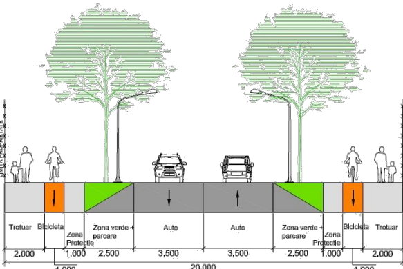
Profil Transversal 16 -lăţime 20m
