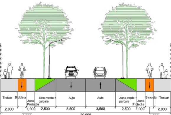
Profil Transversal 16 - lățime 20m
