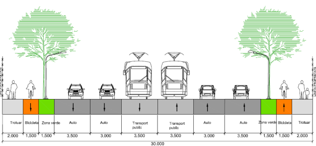
Profil Transversal 55 -lățime 30m
