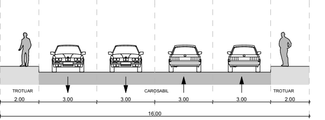
Profil Transversal A - lățime 16m
