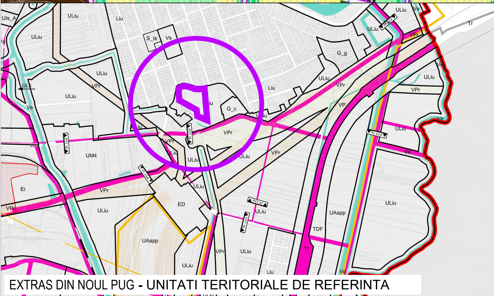
EXTRAS DIN NOUL PUG - ZONIFICAREA PROPUSA
