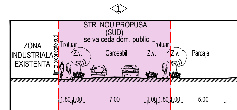
PROFIL TRANSVERSAL STR. PROPUSA (SUD) SC. 1:200
