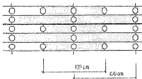
Fixarea lamelor din vată minerală cu diblu cu rozetă suplimentară
