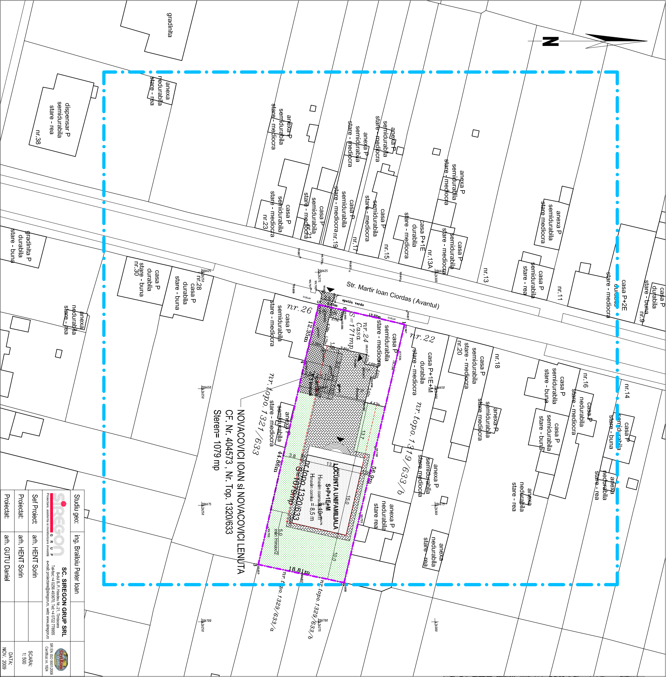
PLAN DE INCADRARE IN LOCALITATE 1:5000
