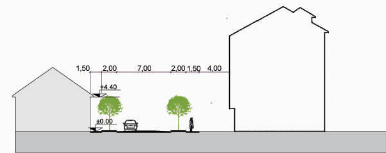
STRADA LETEA - PROFIL EXISTENT SC 1:500
