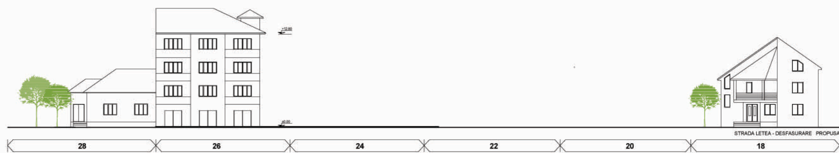
STRADA LETEA - DESFASURARE EXISTENTA SC 1:500
