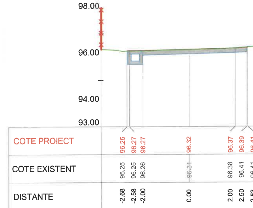
Km 0+040 Profil P2
