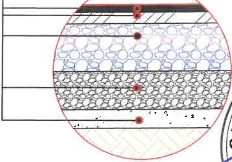
Detaliu A sc. 1:20
