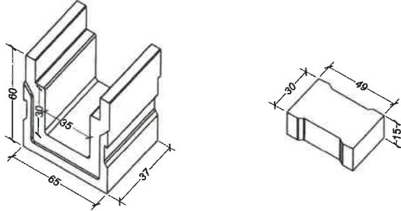
Detaliu C sc. 1:20
