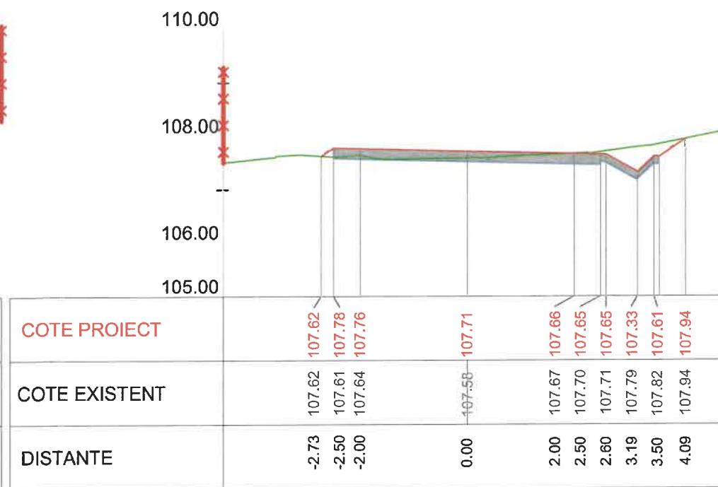
Km 0+300 Profil P14
