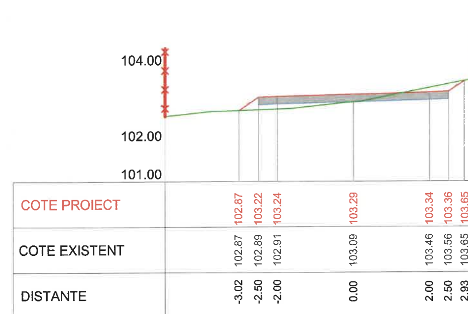
Km 0+120 Profil P6
