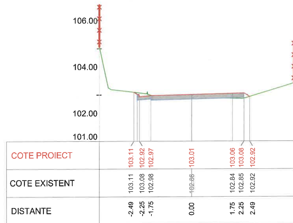
Km 0+260 Profil P13
