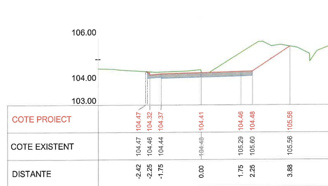
Km 0+200 Profil P10
