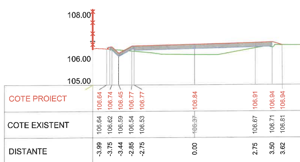
Km 0+140 Profil P7
