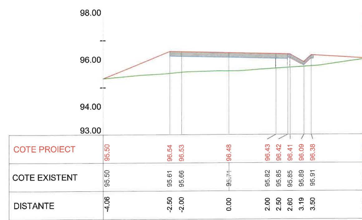
Km 0+820 Profil P38
