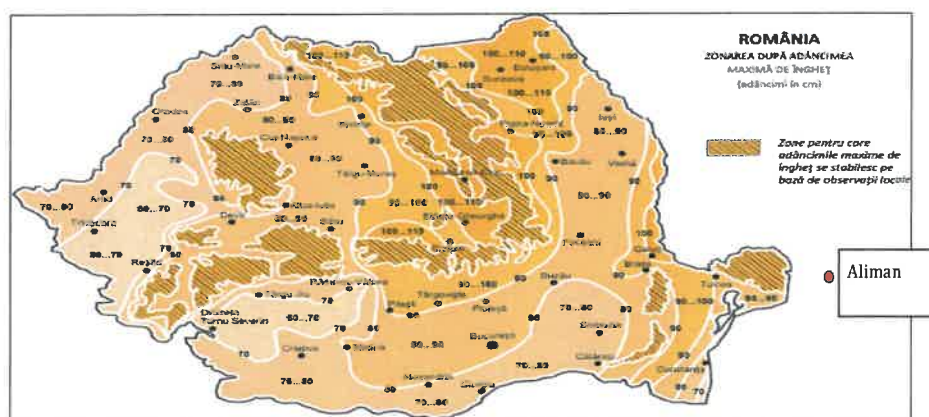
Figura 12 - Adancimea de inghet pe teritoriul Romaniei, conform STAS 6054/1977
