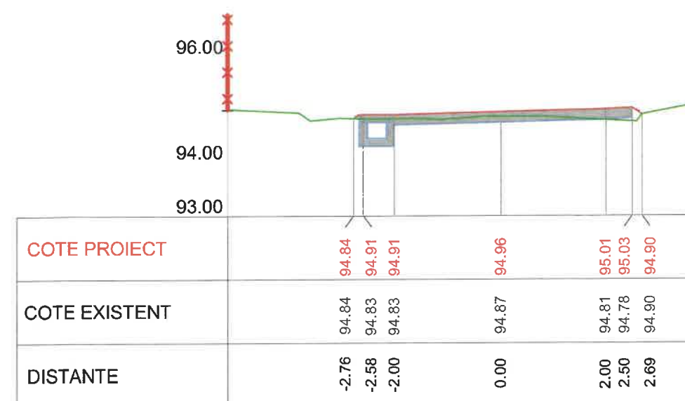
Km 0+120 Profil P6
