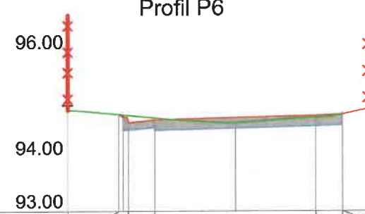
Km 0+120 Profil P6
