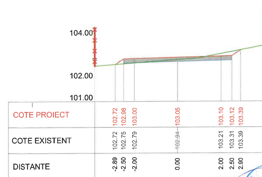
Km 0+160 Profil P8
