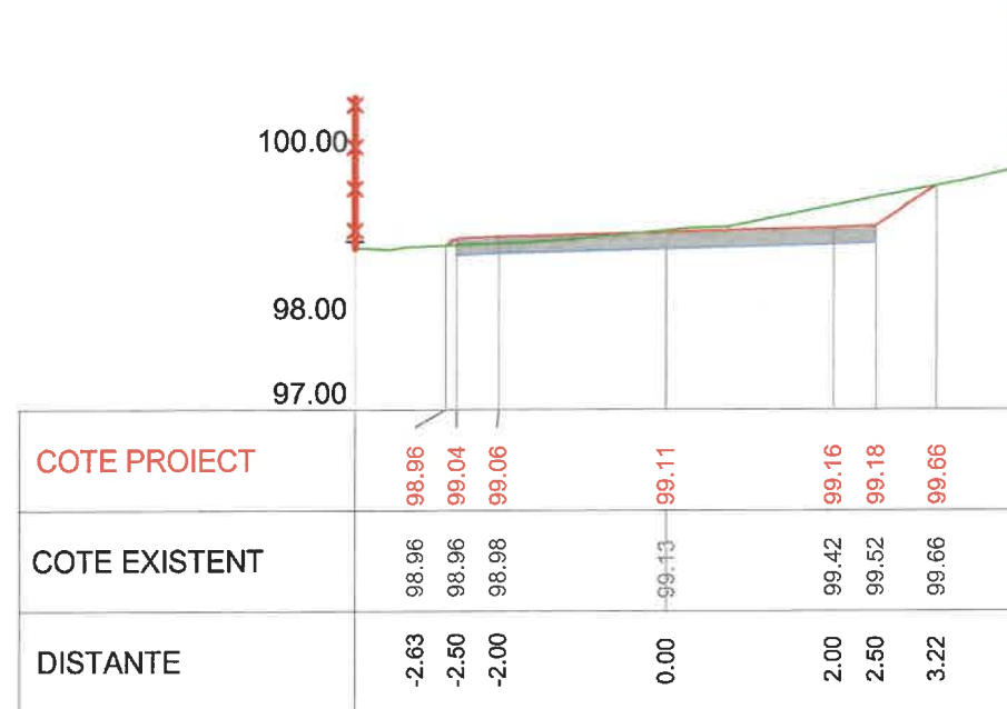
Km 0+340 Profil P17
