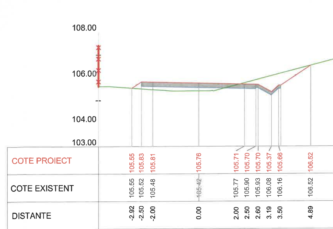
Km 0+380 Profil P18
