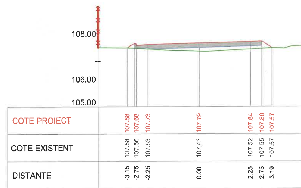
Km 0+040 Profil P2
