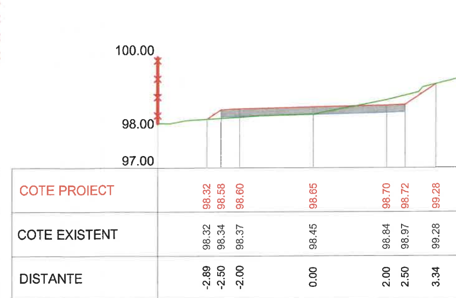
Km 0+360 Profil P18
