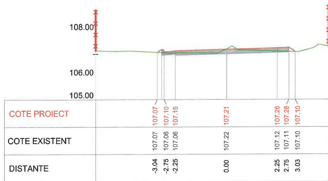
Km 0+020 Profil P1
