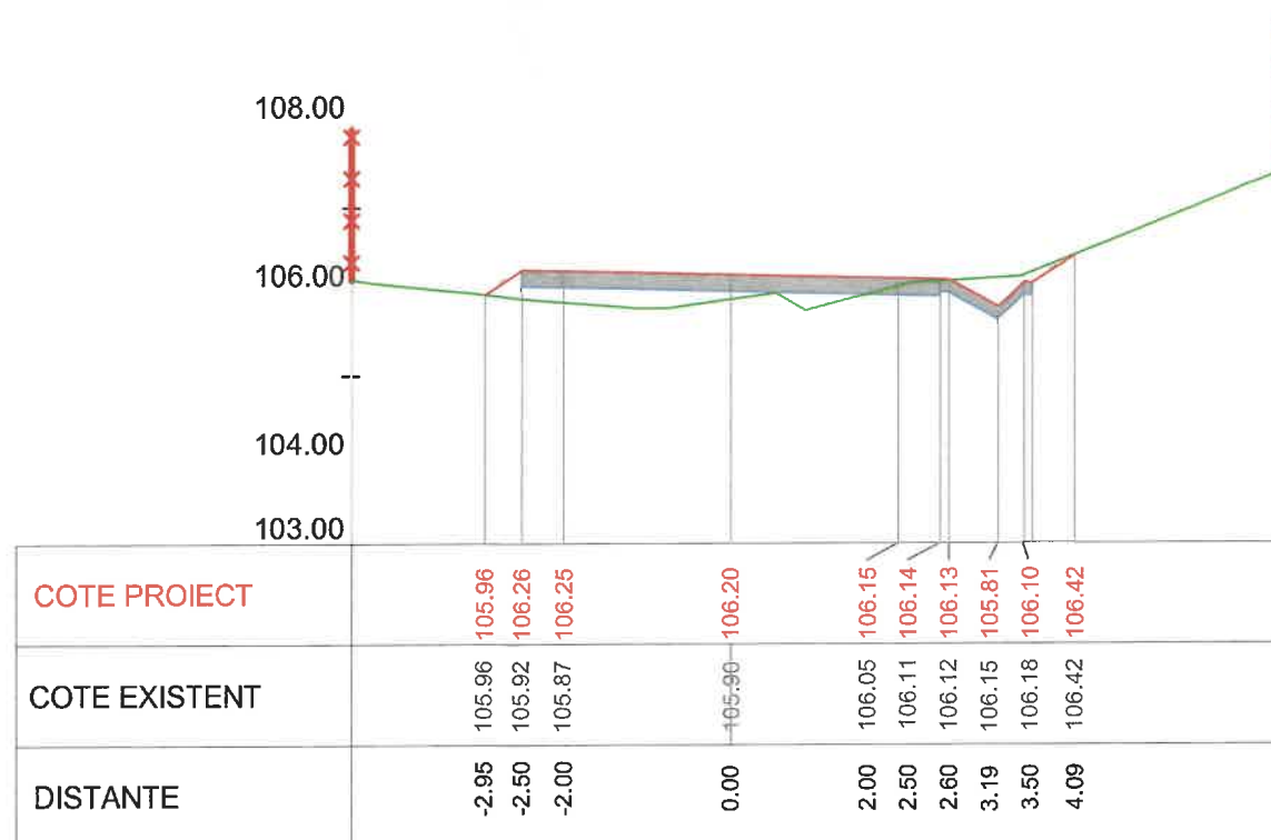
Km 0+360 Profil P17
