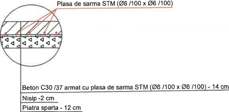
DETALIU SISTEM RUTIER ACCES PROPRIETATI SCARA 1:20
