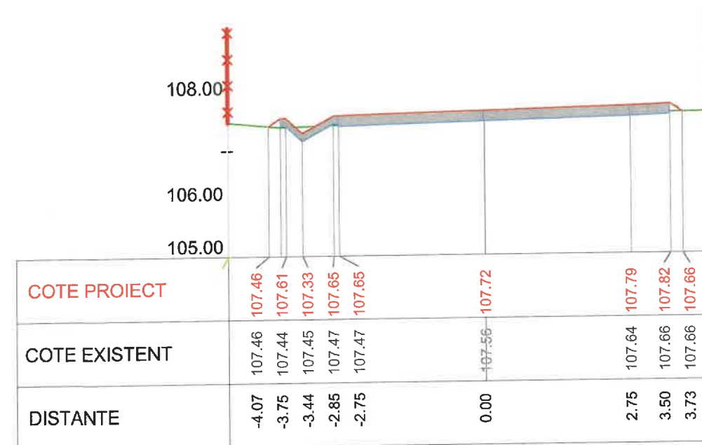
Km 0+080 Profil P4
