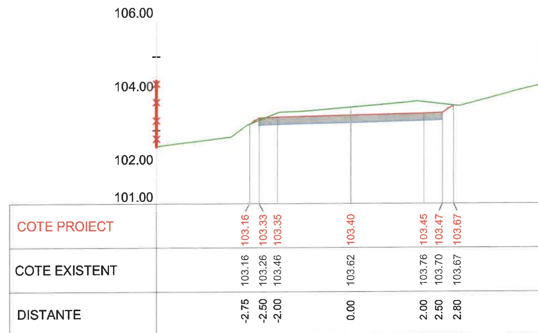
Km 0+100 Profil P5
