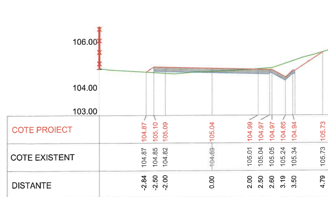
Km 0+420 Profil P20
