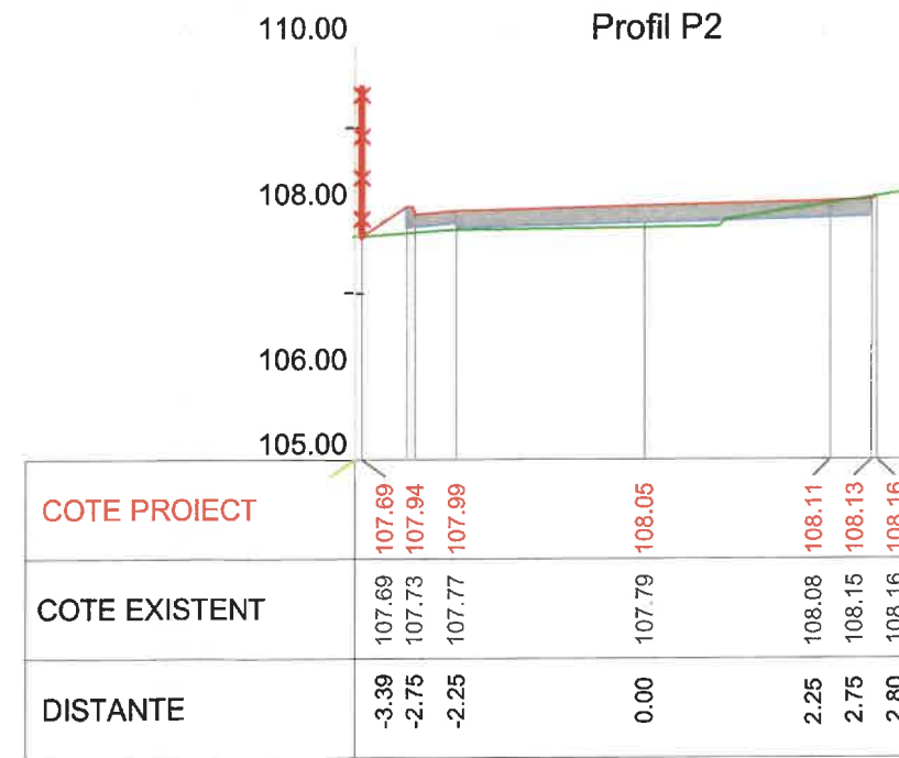
Km 0+080 Profil P4
