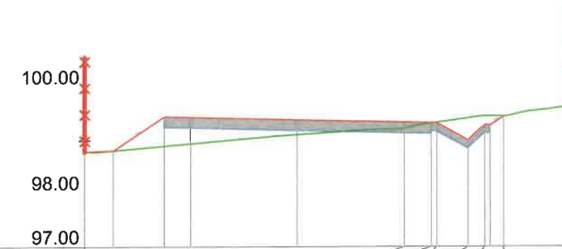
Km 0+560 Profil P26
