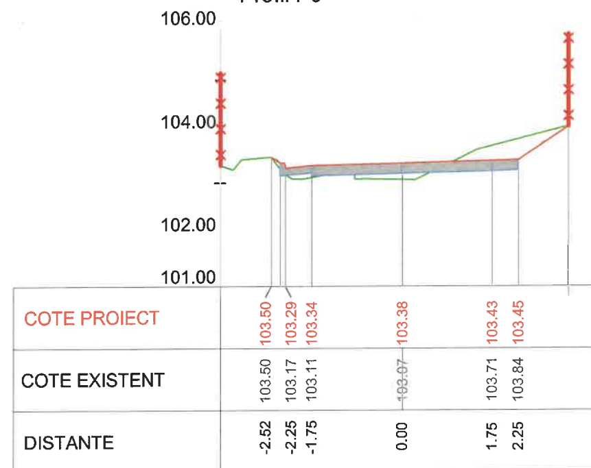
Km 0+220 Profil P11
