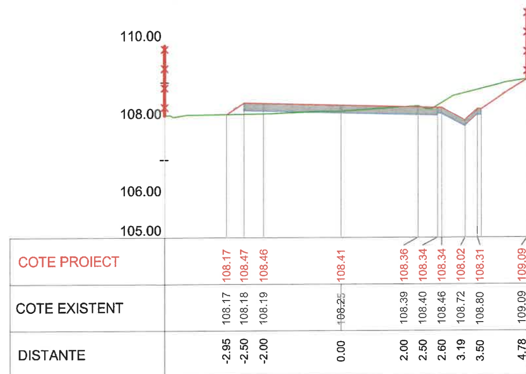
Km 0+040 Profil P2
