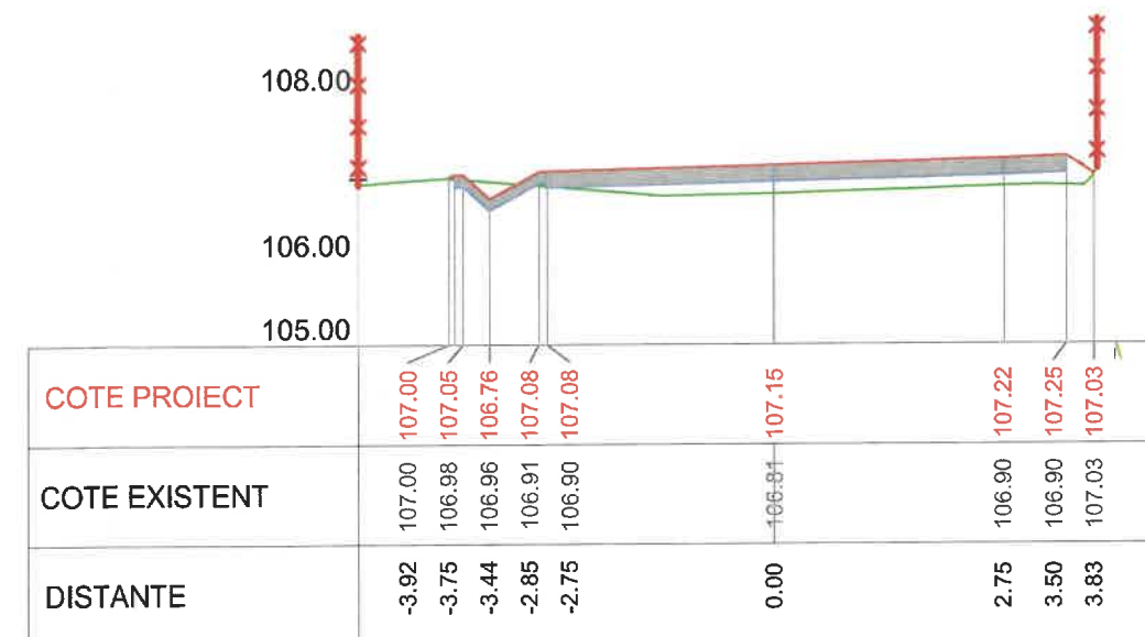
Km 0+120 Profil P6
