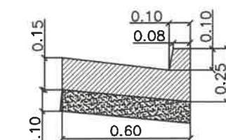
Detaliu C sc. 1:20
