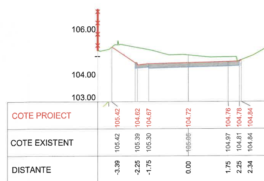
Km 0+280 Profil P14
