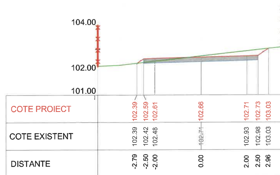
Km 0+180 Profil P9
