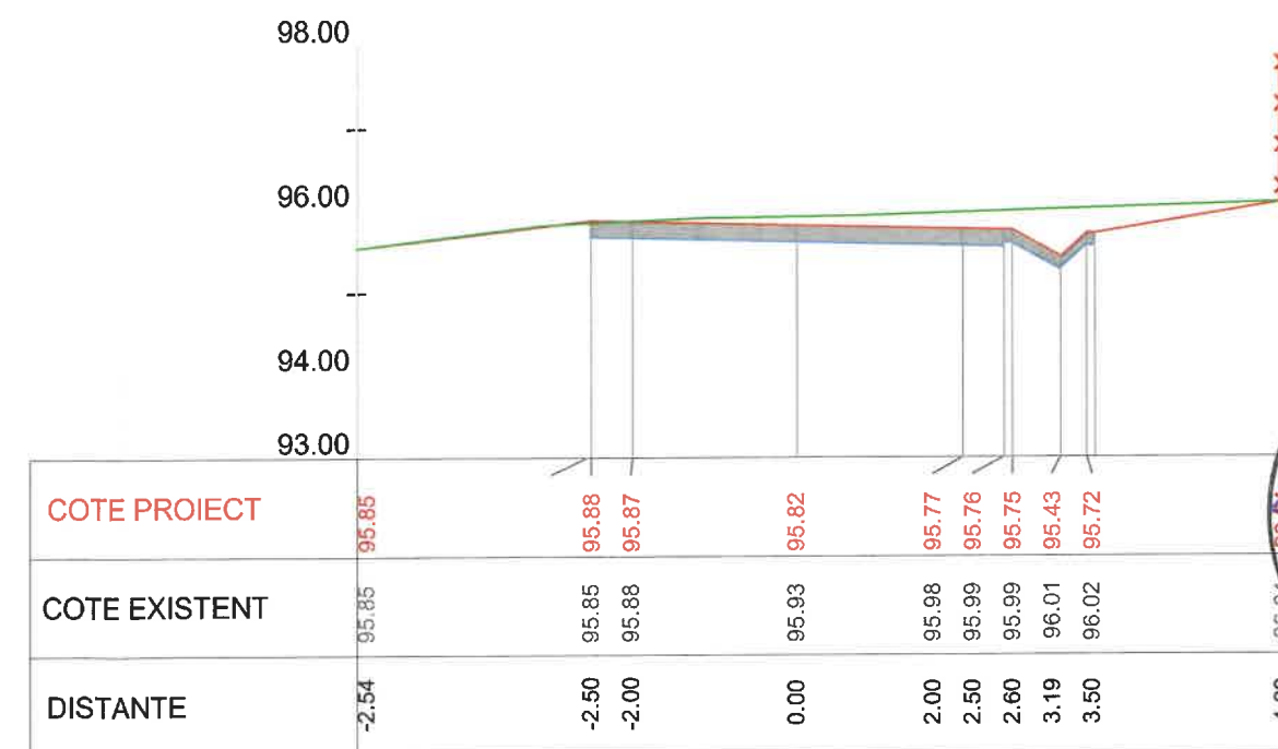
Km 0+860 Profil P40
