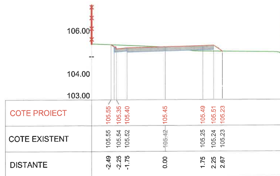
Km 0+180 Profil P9
