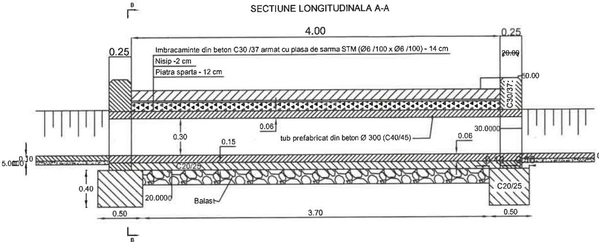
DETALIU SISTEM RUTIER ACCES PROPRIETATI SCARA 1:20
