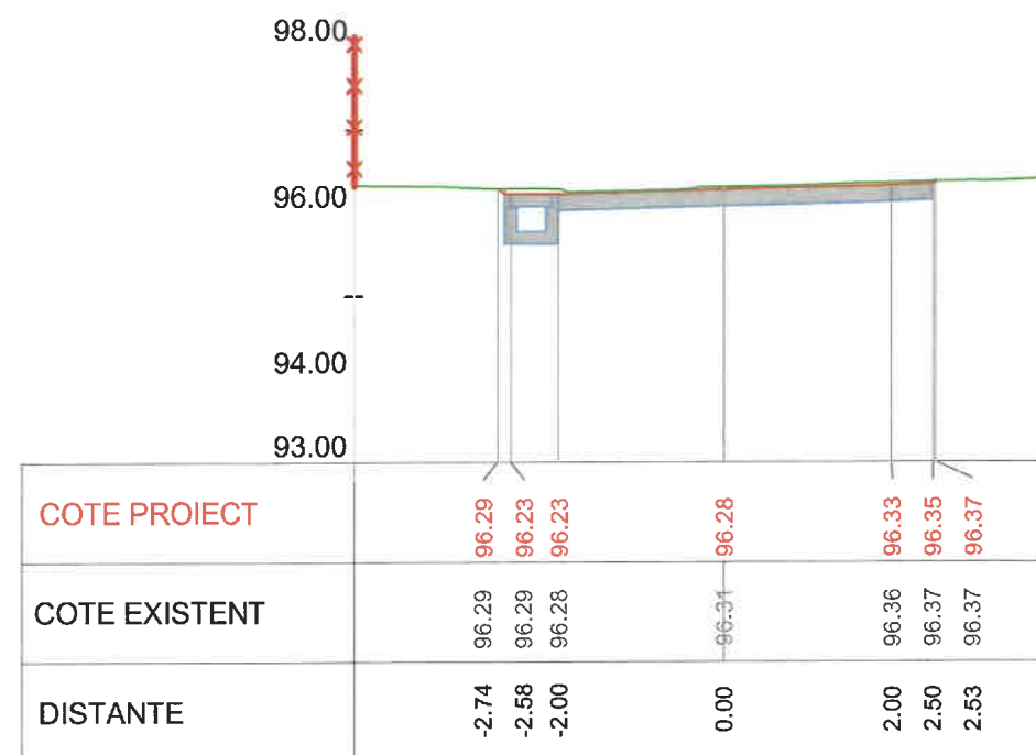
Km 0+020 Profil P1
