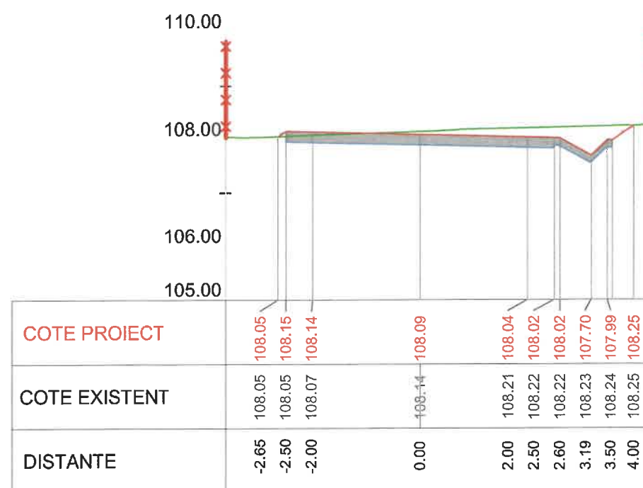
Km 0+280 Profil P13
