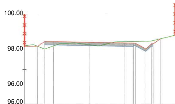
Km 0+640 Profil P29
