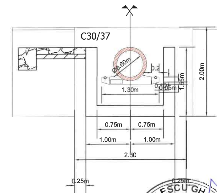
SECTIUNE D - D
