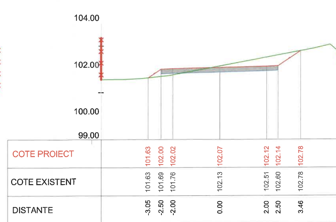
Km 0+200 Profil P10
