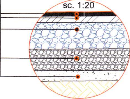
Detaliu A sc. 1:20
