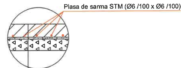
DETALIU SISTEM RUTIER ACCES PROPRIETATI
