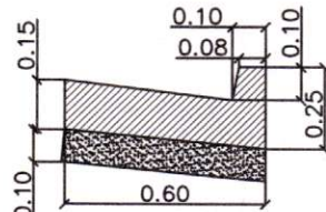
Detaliu C sc. 1:20
