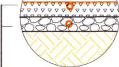
Detaliu B sc. 1:20
