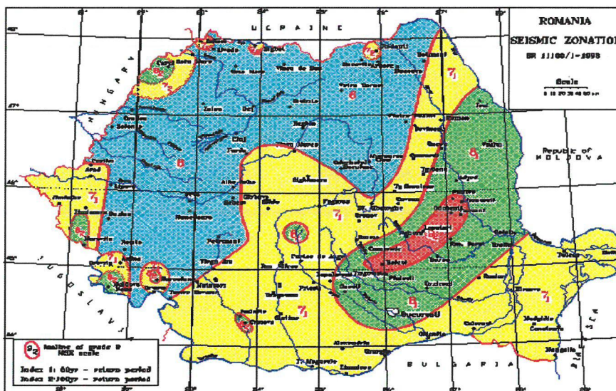
Fig.2. Zonarea seismica
