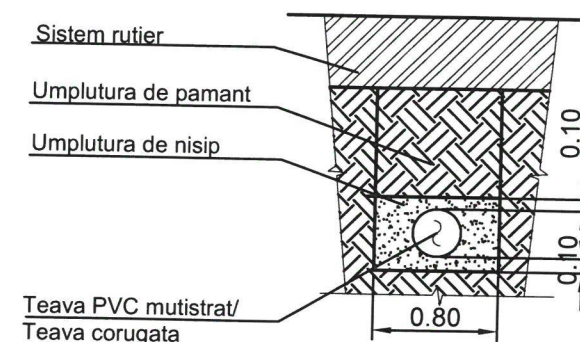
Detaliu de executie sant pentru conducta de canalizare
