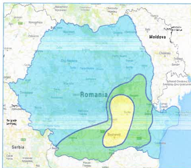
Zonarea teritoriului în termeni de valori de vârf ale accelerației terenului pentru proiectare ag. și în termeni de perioada de control (coll), Tc, a spectrului de raspuns
