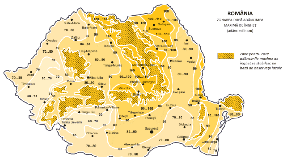
Fig. 6 - Zonarea teritoriului României după adâncimea de îngheț, conform STAS 6054 / 77. Adâncimi maxime de îngheț
