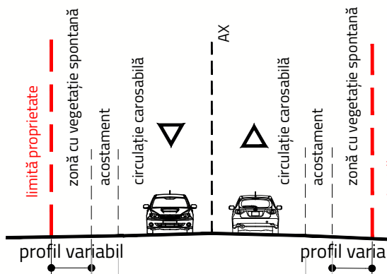
PROFIL TRANSVERSAL AA' - DN2A Profil existent
