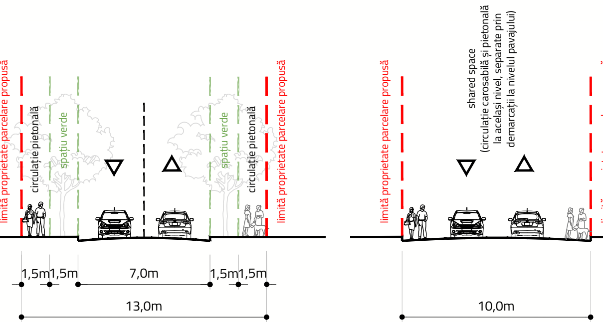
PROFIL TRANSVERSAL BB' Profil propus
