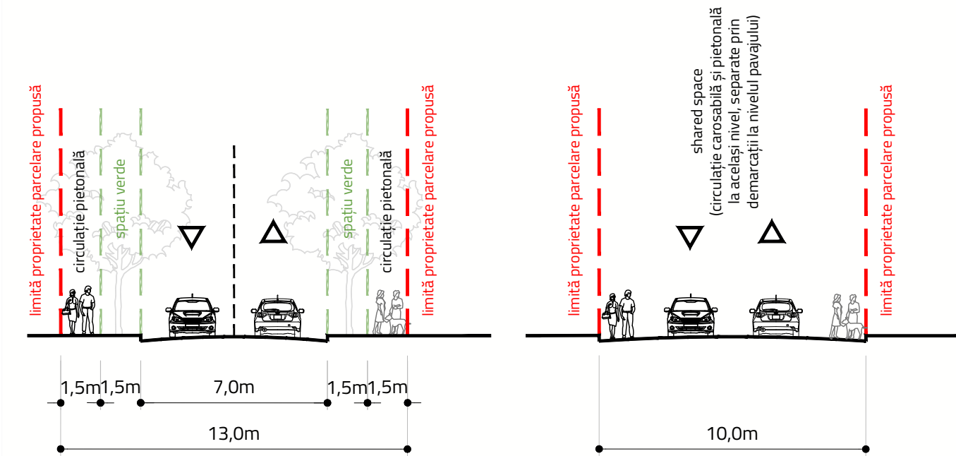
PROFIL TRANSVERSAL BB' Profil propus
