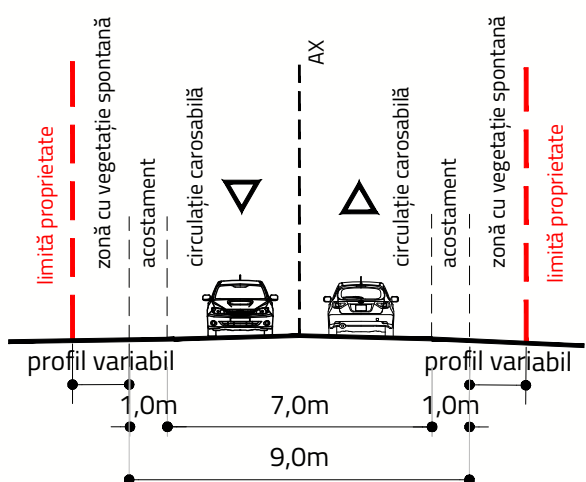
PROFIL TRANSVERSAL AA' - DN2A Profil existent
