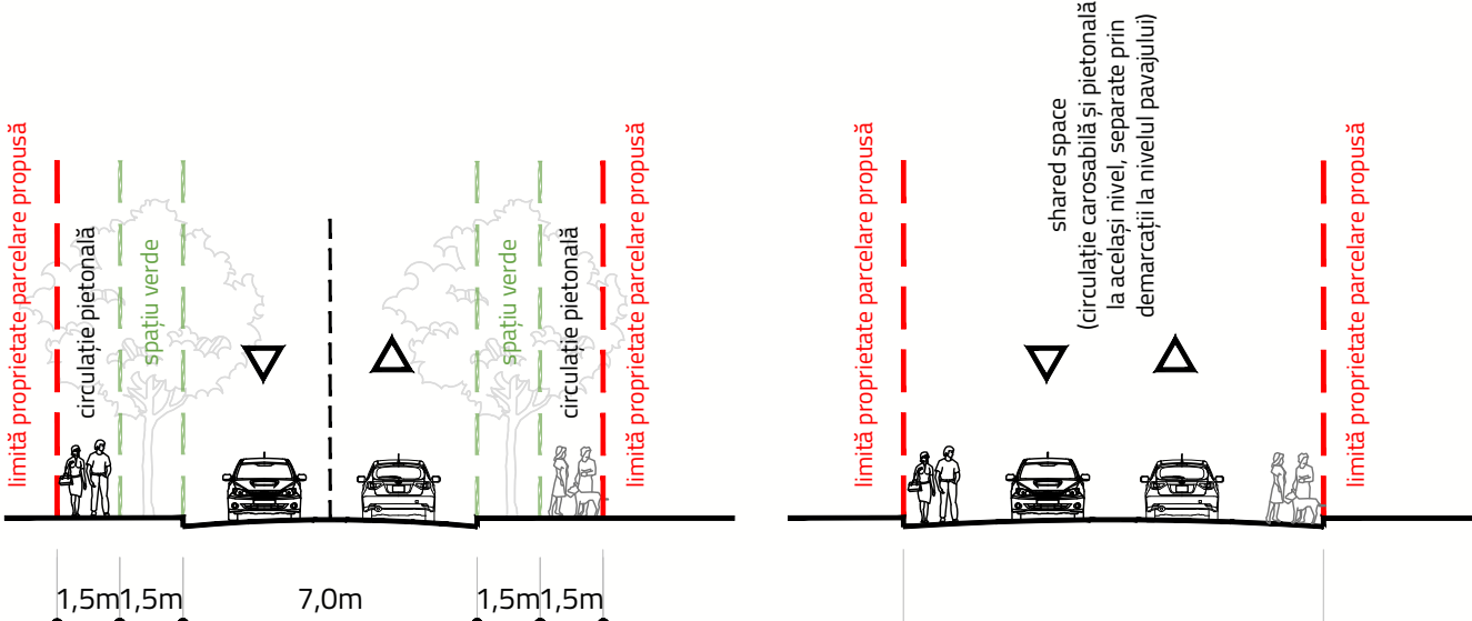
PROFIL TRANSVERSAL BB' - Profil propus
