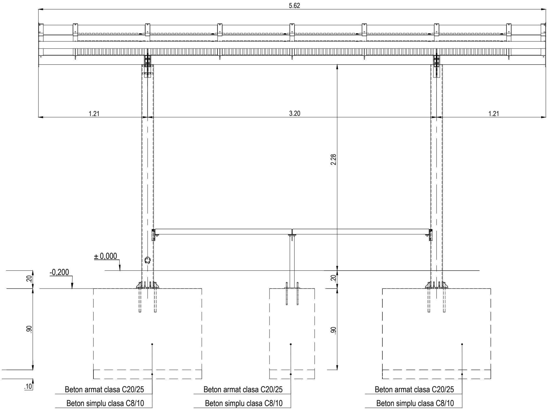
SECTIUNE LONGITUDINALA
