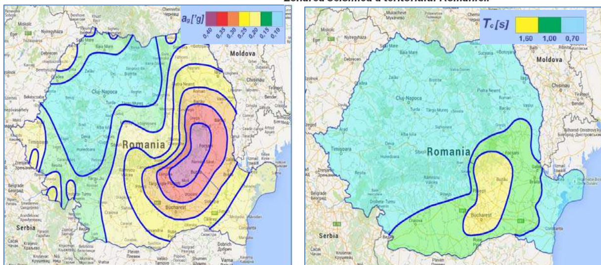
Zonarea teritoriului în termeni de valori de varf ale accelerației terenului pentru proiectare a_g și în termeni de perioadă de control (colț), T_c , a spectrului de răspuns
