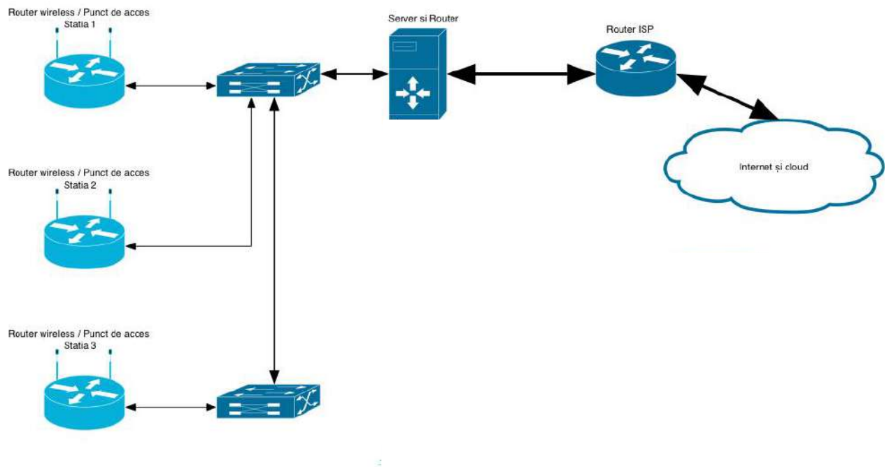
Fig. 3.5. Structura sistemului de acces la Internet
