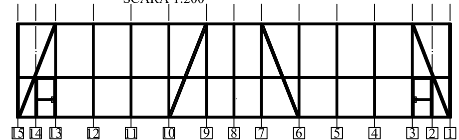
FAȚADĂ EST - TEREN MULTIFUNCȚIONAL BULEVARDUL 1 DECEMBRIE SCARA 1:200
