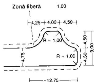
④ Întoarcere în formă de T pentru autoturisme
