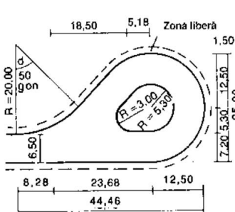
⑧ Bucă de întoarcere pentru camioanele grele și autobuzele articulate
