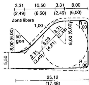
⑨ Cerc de viraj pentru mașinile de gunoi cu 2 osii resp. pentru autocamioane de 6 m
