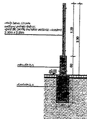
SECȚIUNE VERTICALĂ 3
