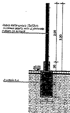
SECȚIUNE VERTICALĂ 2
