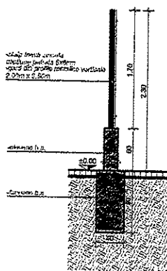
SECȚIUNE VERTICALĂ 1
