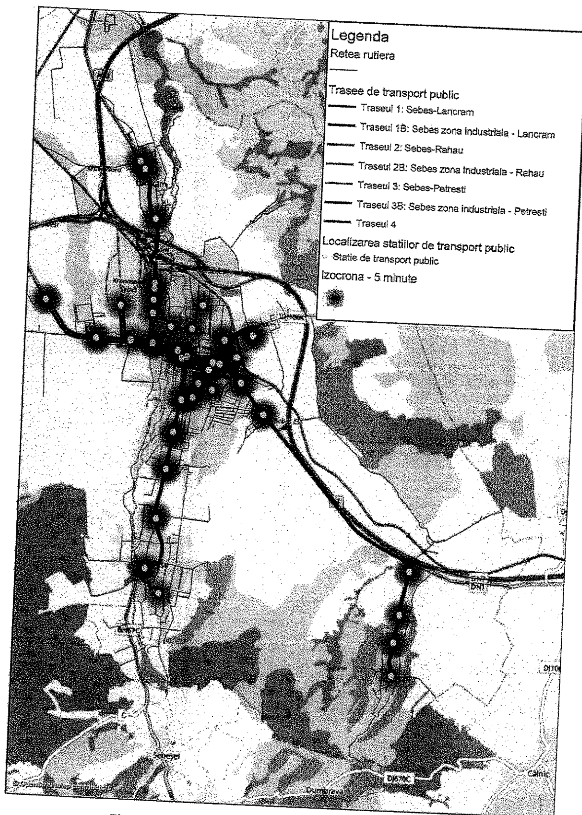
Figura 3.1. Traseele de transport public și stațiile propuse.
