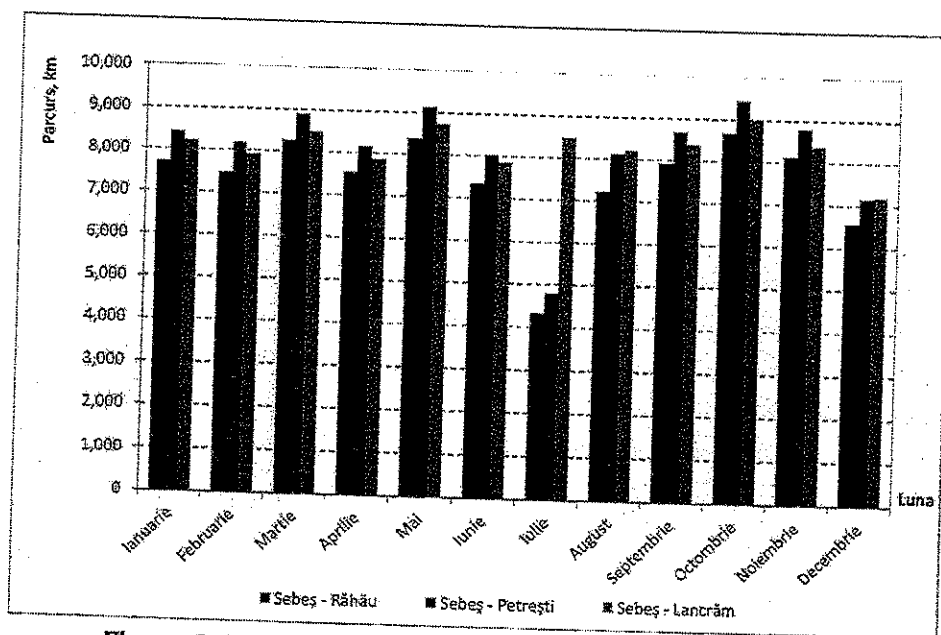
Figura 2.18. Parcursul lunar al mijloacelor de transport, 2019.
