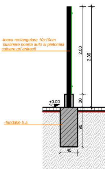
SECȚIUNE VERTICALĂ 2
