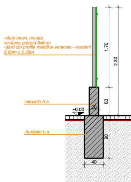
SECȚIUNE VERTICALĂ 3
