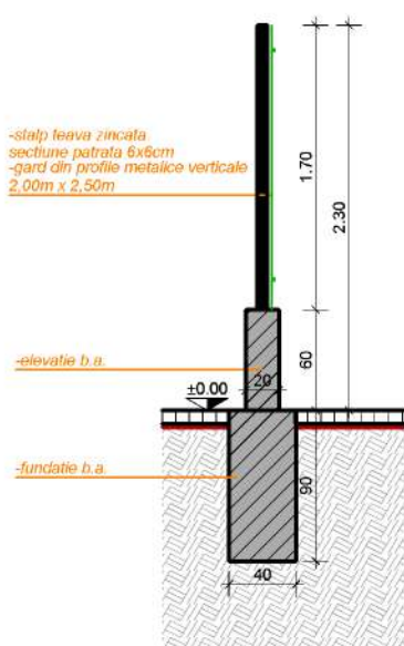
SECȚIUNE VERTICALĂ 1
