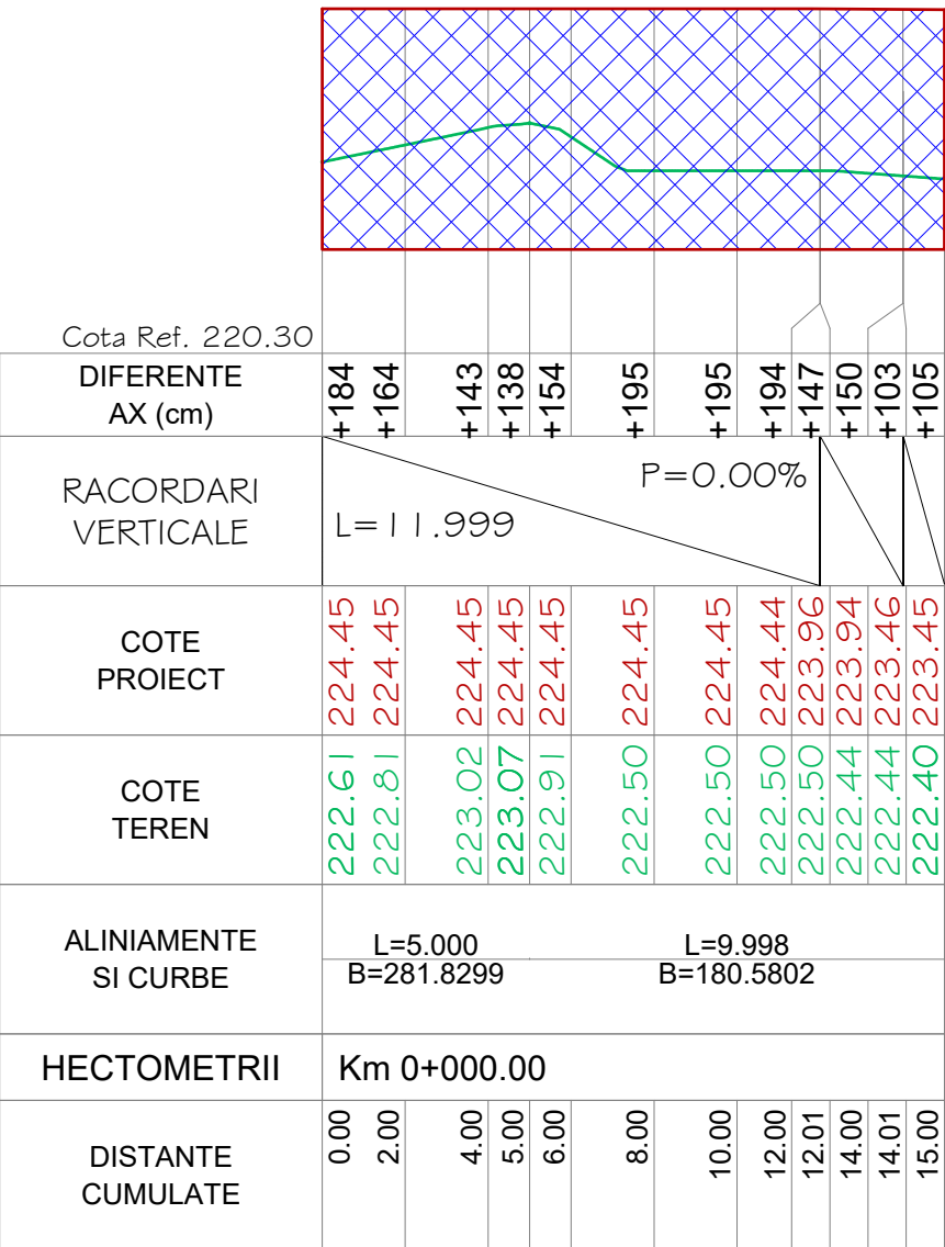
PROFIL LONGITUDINAL ZID_2 DE LA 0.000 LA 14.998 SCARA : ORIZ 1 :200 VERT 1 :100
