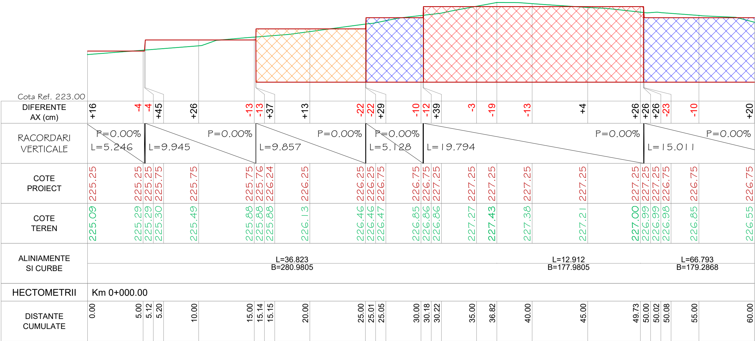
PROFIL LONGITUDINAL zid DE LA 0.000 LA 60.000 SCARA : ORIZ 1 :200 VERT 1 :100
