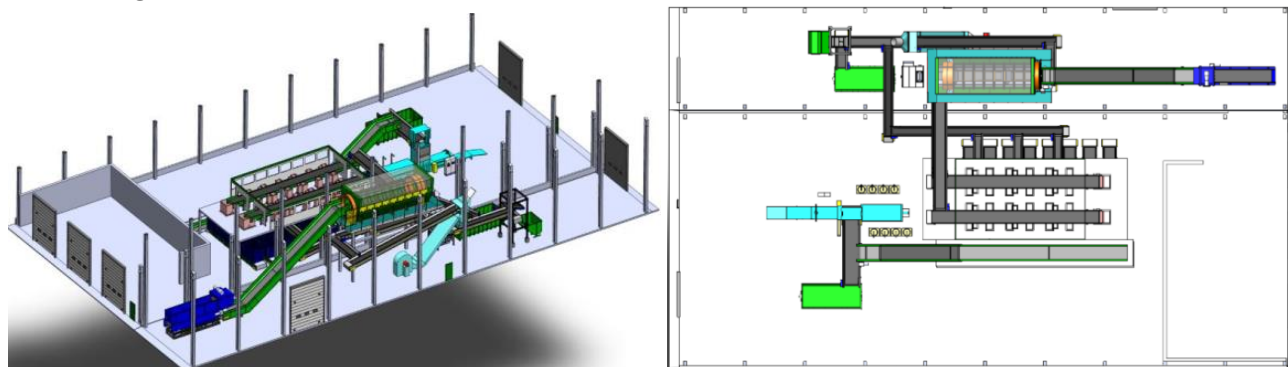
Figură 3-53 Perspectivă și vedere de sus a liniei de sortare hârtie/carton propuse
