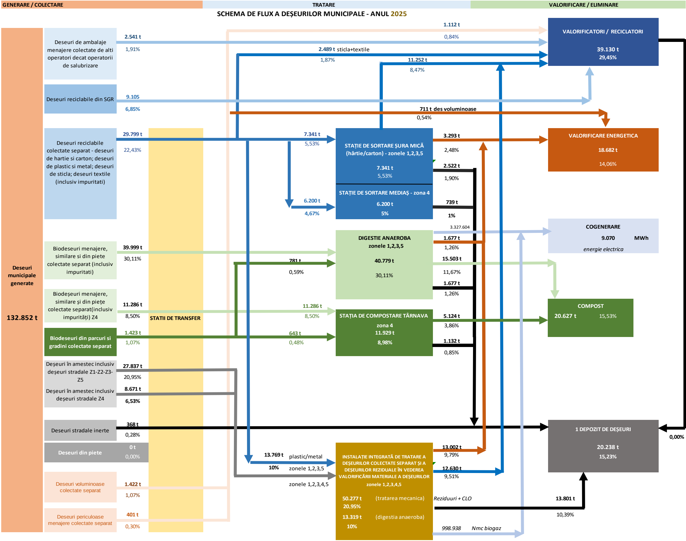
Figură 3-15 Alternativa 2 - Schema flux deșeurilor municipale - anul 2025
