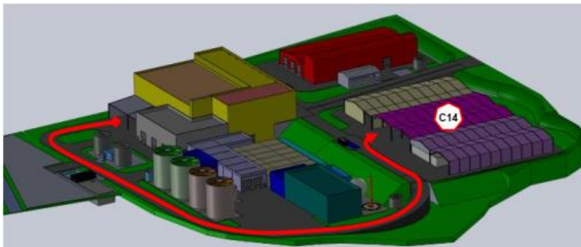
Figură 3-60 Transferul baloților către Hala C14
