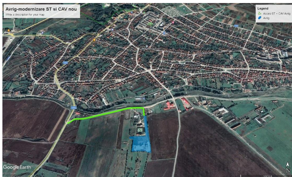
Figură 3-30 CAV Avrig – plan amplasament
