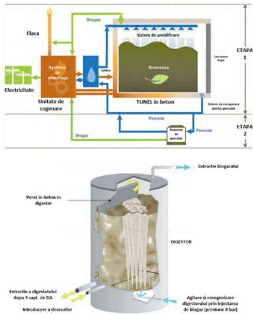
Figură 3-7 – Digestie anaerobă uscată (exemple)
