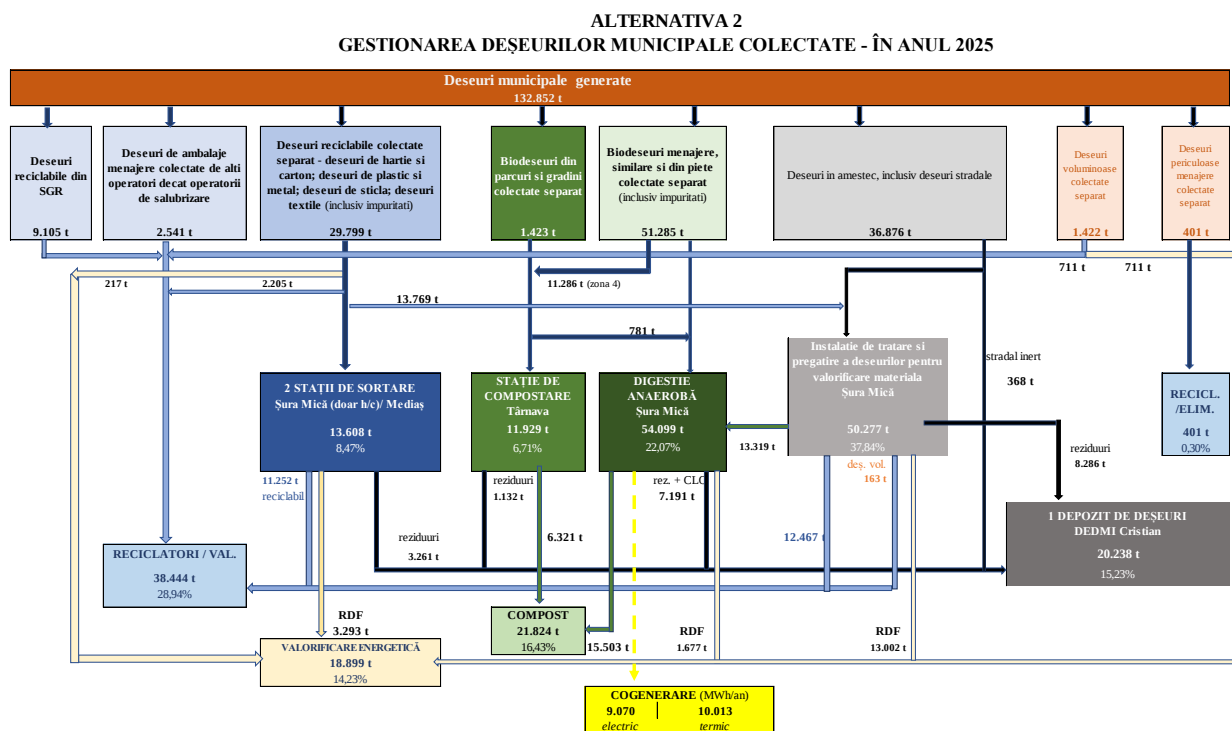
Figură 5-1 Schema flux deșeuri municipale - anul 2025
