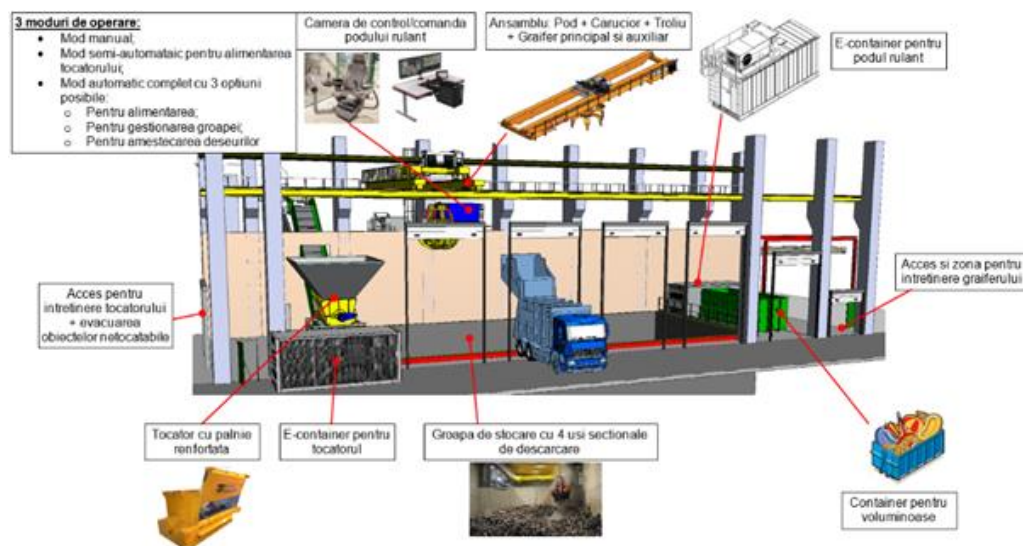
Figură 3-50 TMB cu bioscări – exemplu recepție groapă cu pod rulant și graifer
