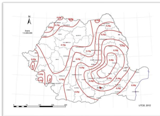
Zona seismică a teritoriului României.
