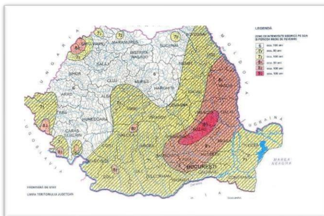
Zona seismică a teritoriului României.
