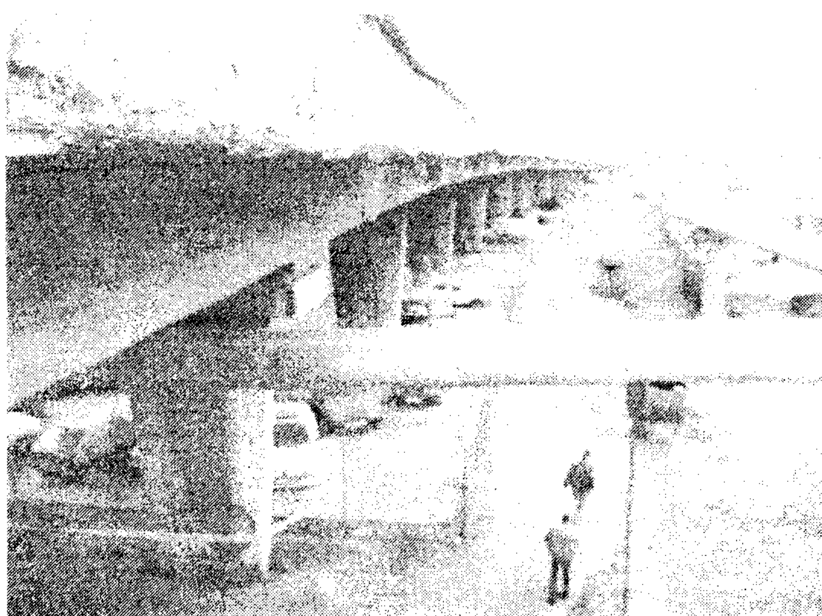
Fotografia 6 Degradări beton și armatura în grinda de parapet, generalizate pe toată lungimea pasajului
