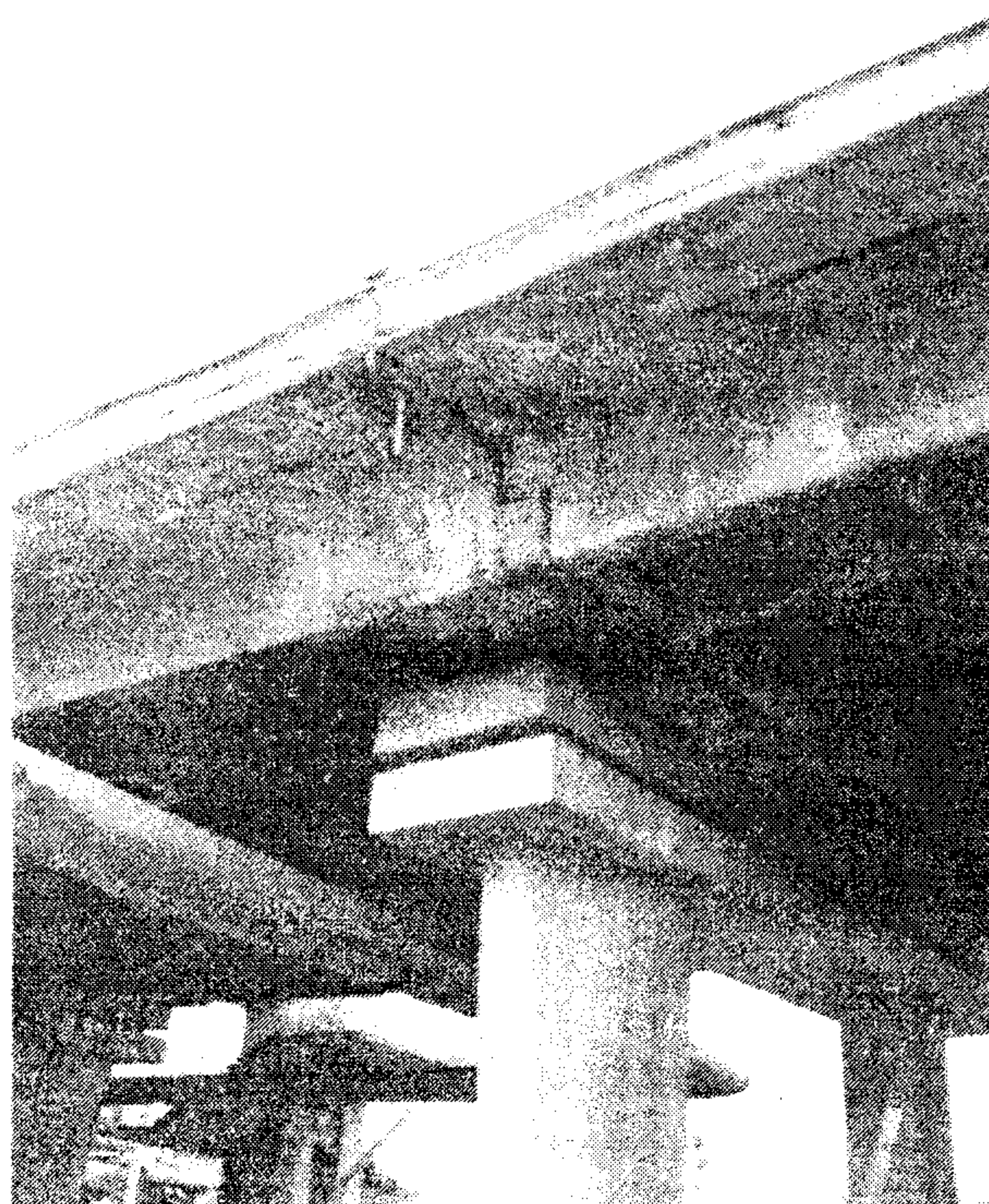
Fotografia 3. Degradări cauzate de infiltrații în rostul Gerber Pila P12
