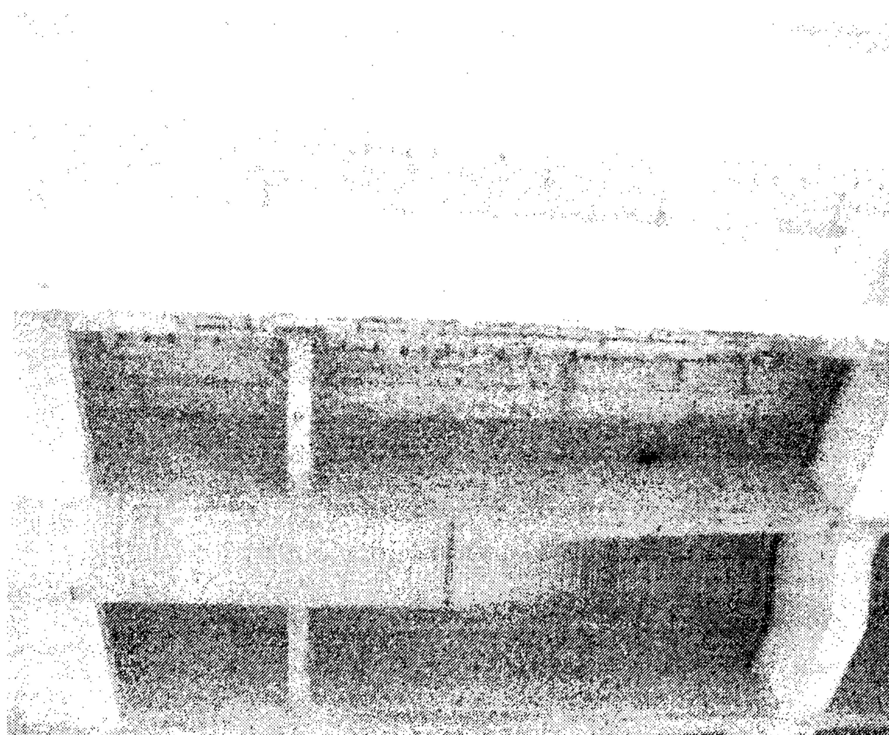
Fotografia 5 Degradări importante în betonul și armatura structurii de rezistență a tablierului.
