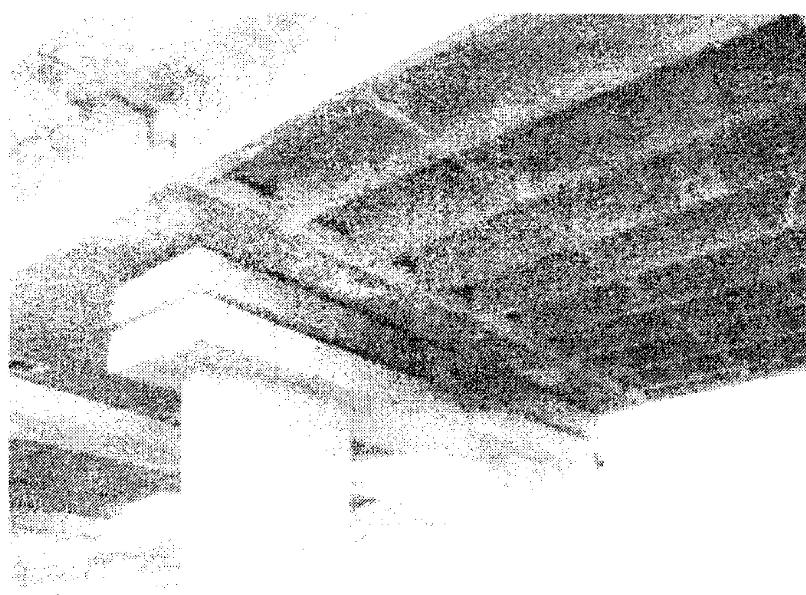
Fotografia 4. Degradări cauzate de infiltrații în rostul Gerber Pila P1
