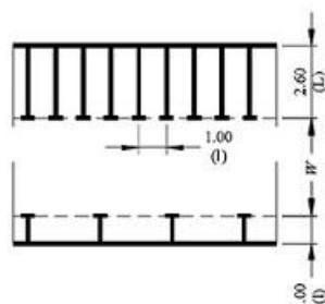
Figura 6.4 Parcare mototocicletelor la 90° și longitudinal
