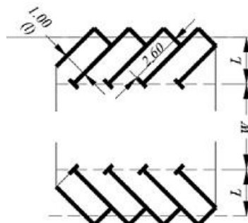
Figura 6.5 Parcare mototocicletelor la 45°
