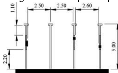
Figura 5.3 Parcarea la 90° alăturată elementelor de construcție poziționate la o distanță cuprinsă între 1.10 m și 2.80 m față de marginea căii de circulație
