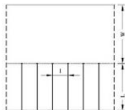
Figura 6.6 Parcare la 90^\circ
