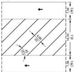
Figura 6.8 Parcare autovehiculelor articulate la 45^\circ
