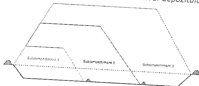
Figura 1 Configurația Celulei 1 din cadrul depozitului Țuțora
