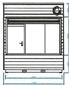
Fațadă principală - ușa deschisă
