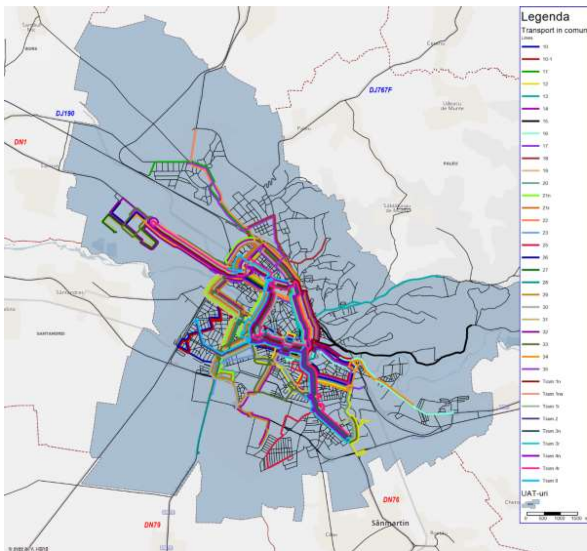
Figură o-5 Harta liniilor de transport în comun – municipiul Oradea
