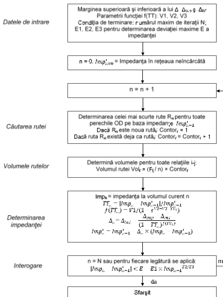
Figură 0-11 Schema logică a metodei "Echilibru-Lohse" de afectare pe itinerarii
