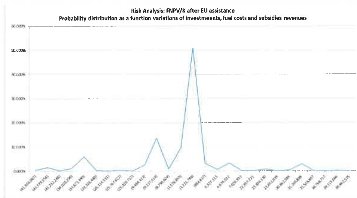
Figura 4 – Distribuția probabilității VNAF/K
