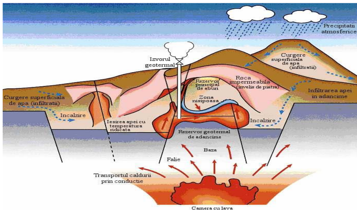
Structura unui sistem geotermal ideal
