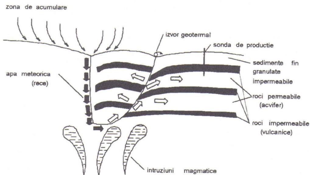
Zăcăminte de entalpie scăzută în bazin sedimentar
