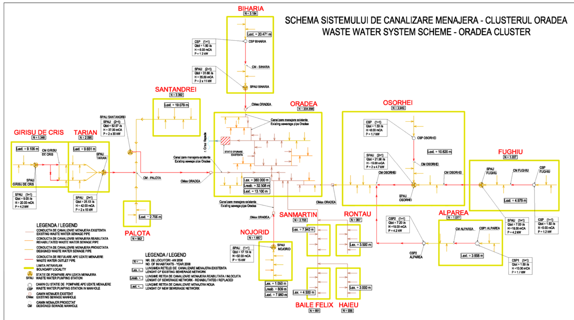
Figura4-3 Schema sistemului propus pentru canalizarea menajera – Clusterul Oradea:
