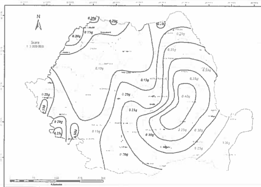
România - Zonarea valorilor de vârf ale accelerației terenului pentru proiectare a_g cu IMR = 225 ani și 10% probabilitate de depășire în 50 de ani
