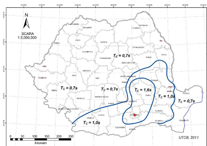
Fig. 4 Zonarea teritoriului Romaniei in termeni de perioada de control (colt), T_c a spectrului de raspuns (P100-1/2013)
