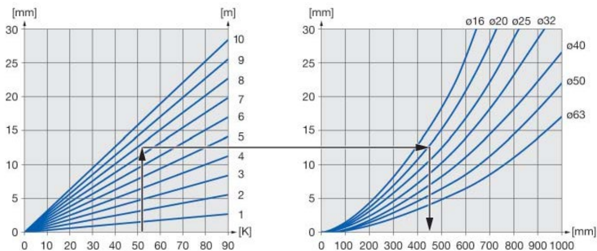
Fig. 1 – 14 Dilatație liniară țevi din PE-Xc
