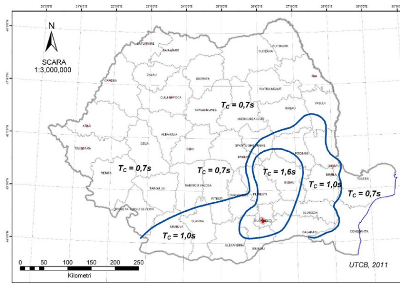
Fig. 5 Zonarea teritoriului Romaniei in termeni de perioada de control (colt), T_c a spectrului de raspuns (P100-1/2013)
