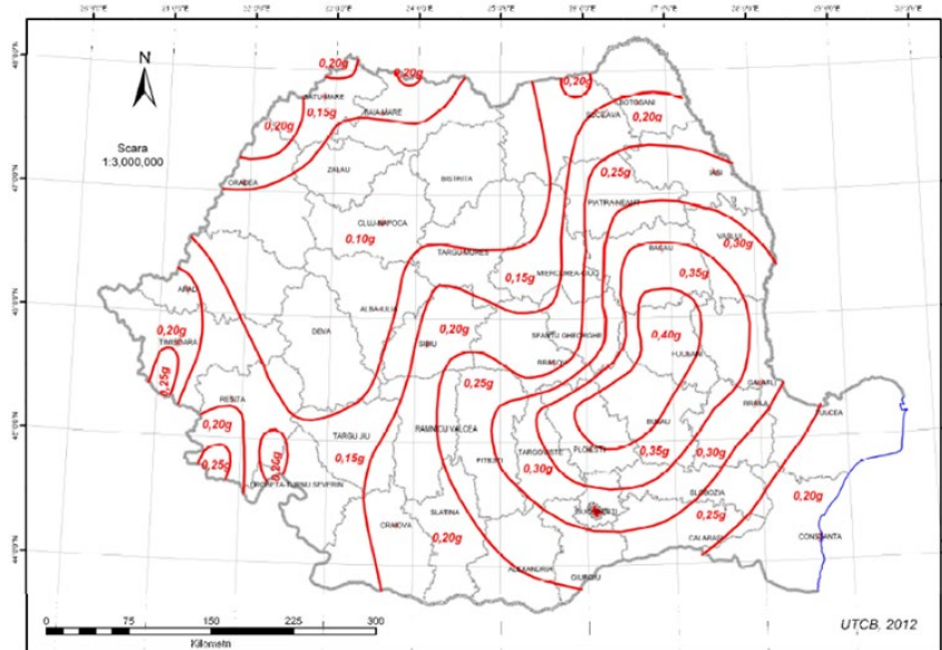
Fig. 4 Zonarea teritoriului Romaniei in termeni de valori de varf ale acceleratiei terenului pentru proiectare, a_g , pentru cutremure avand intervalul mediu de recurenta IMR=225 ani (P100-1/2013)
