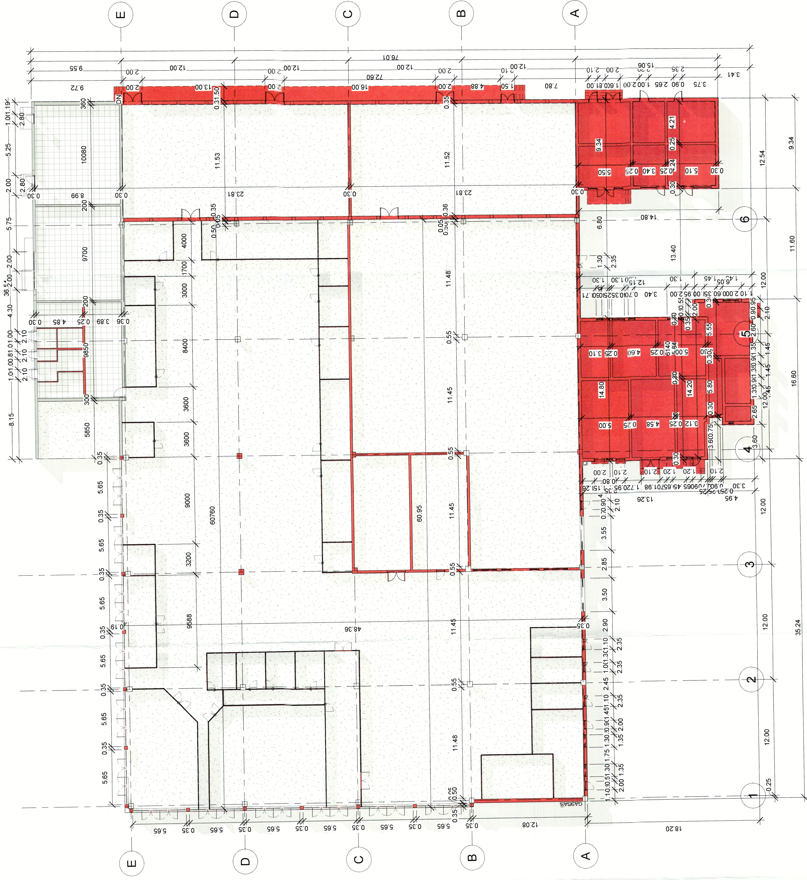
1 Plan Parter Interventii 1 : 200
