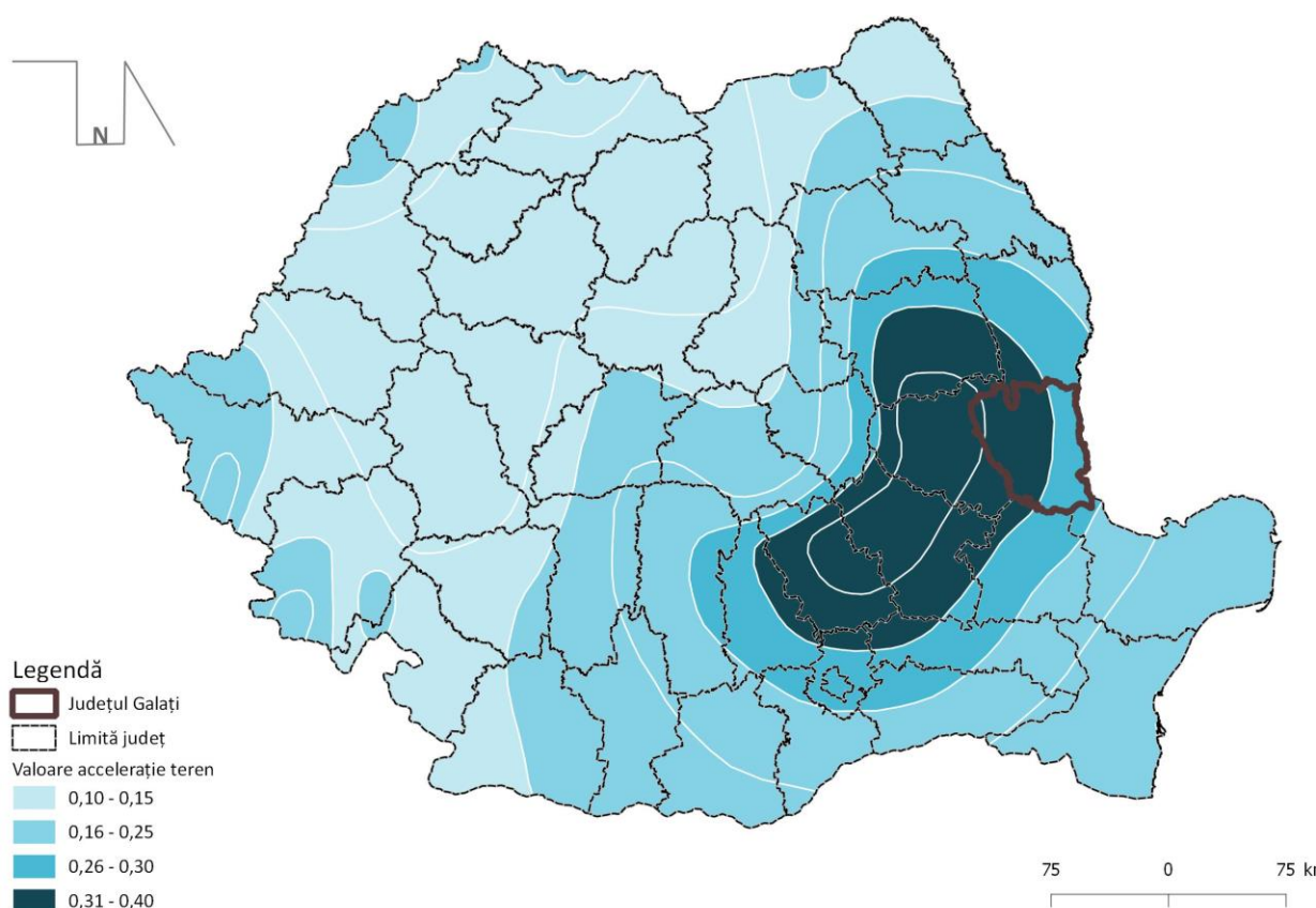
FIGURA 105. VALORILE DE VÂRF ALE ACCELERAȚIEI TERENULUI PENTRU CUTREMURE CU IMR DE 224 ANI (G)
