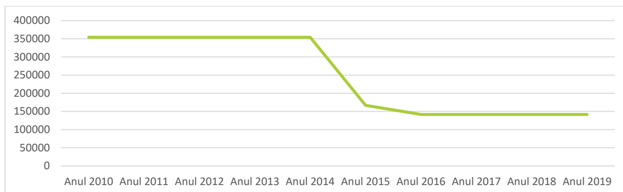
FIGURA 88. CAPACITATEA INSTALAȚIILOR DE PRODUCERE A APEI POTABILE ÎN MUNICIPIUL GALAȚI
