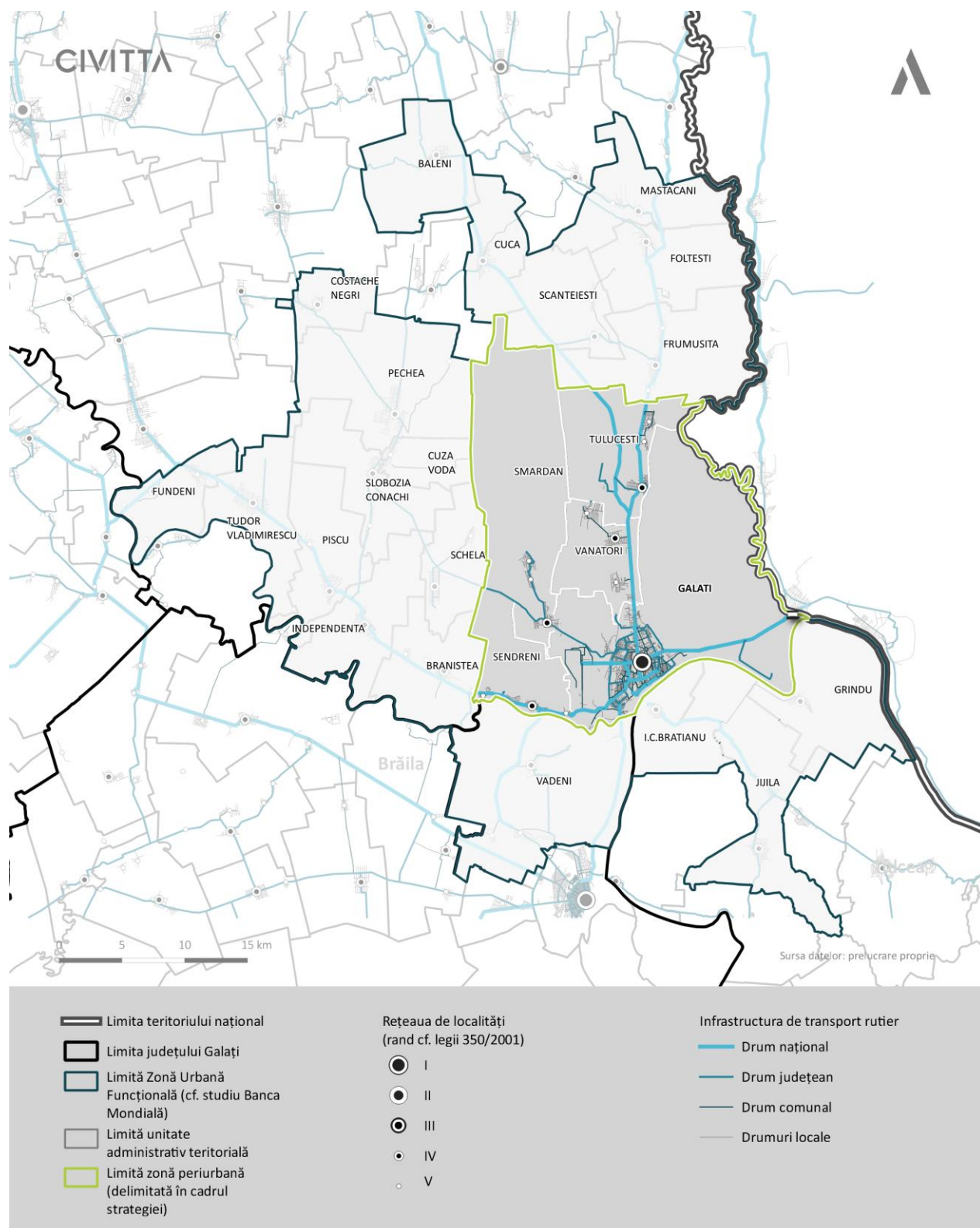
FIGURA 70. REȚEAUA DE DRUMURI DIN MUNICIPIUL GALAȚI ȘI ZONA PERIURBANĂ
