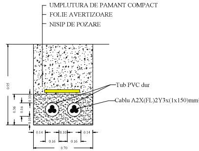
DETALIU PROFIL "M" CABLU MT
