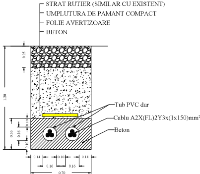
DETALIU PROFIL "T" CABLU MT
