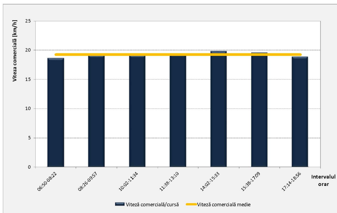
Figura 3.19.b. Variația vitezei comerciale pe Linia 27, 2019.
