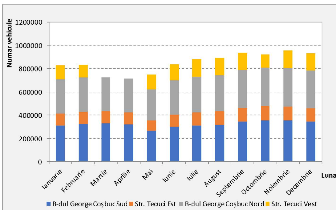
Figura 3.3, a. Variația lunară a volumelor de trafic, intersecția B-dul George Coșbuc – Str. Tecuci, anul 2018.
