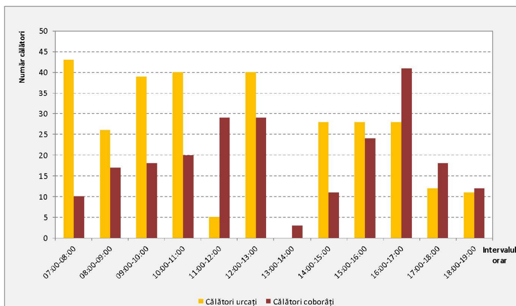
Figura 3.57. Variația orară a fluxurilor de pasageri, Stația "Gara C.F.R."
