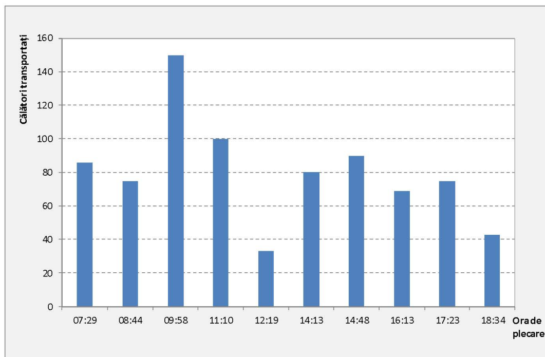
Figura 3.51. Volume de călători/cursă, Linia 104T.
