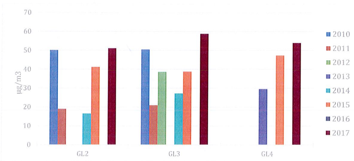
Figura nr. 4-2: Tendința concentrațiilor medii anuale pentru ozon ( \text{O}_3 ) în aglomerarea Galați, între anii 2010-2017
