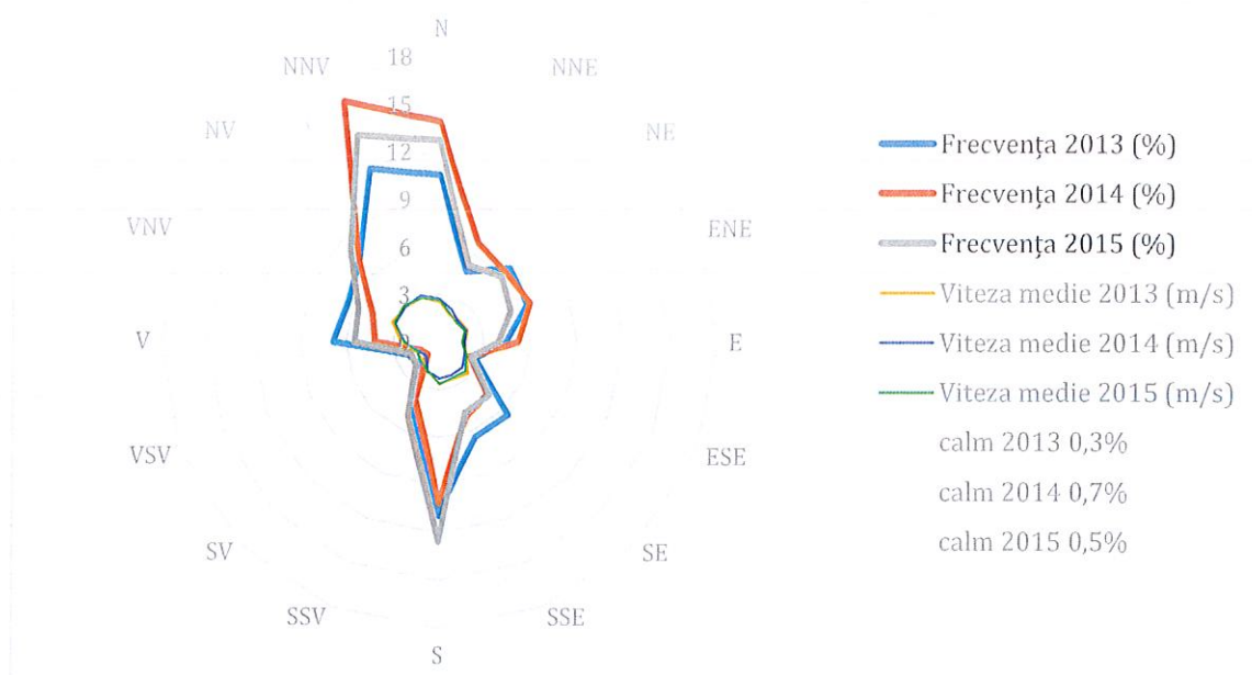
Figura nr. 2-13: Roza vânturilor medii pentru municipiul Galați, 2013-2015
