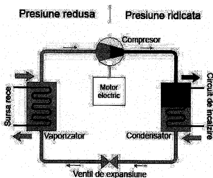
Fig. 2.c - Principiul de funcționare al pompei de căldură
