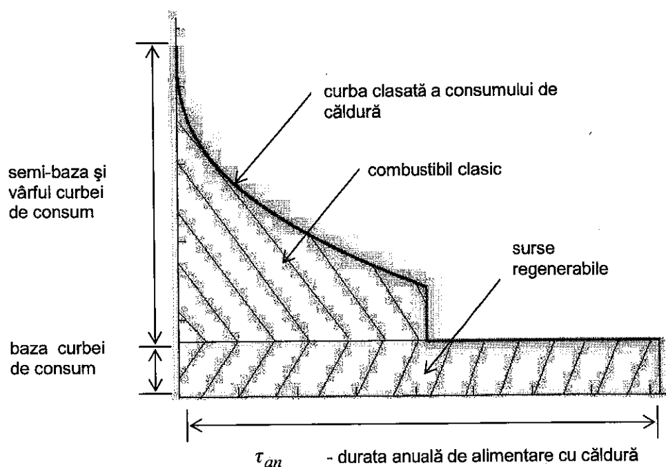
Fig. 2.a – Conceptul de utilizare a surselor regenerabile și combustibililor clasici, pentru asigurarea cererii urbane anuale de căldură a SACC urbane.
