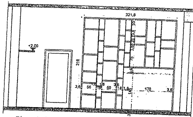
Elevatie interloara E3
