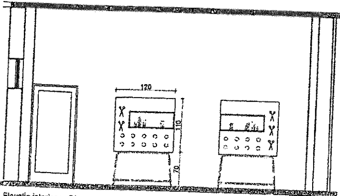
Elevatie interioara C1
