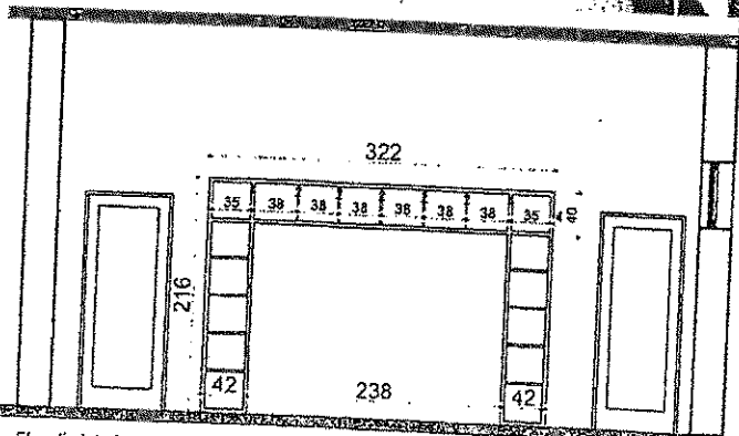
Elevatie interioara C2
