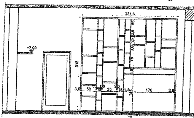
Elevatie interioara E3
