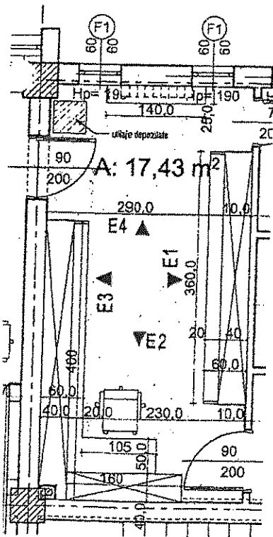
PLAN SALA DE CLASA
