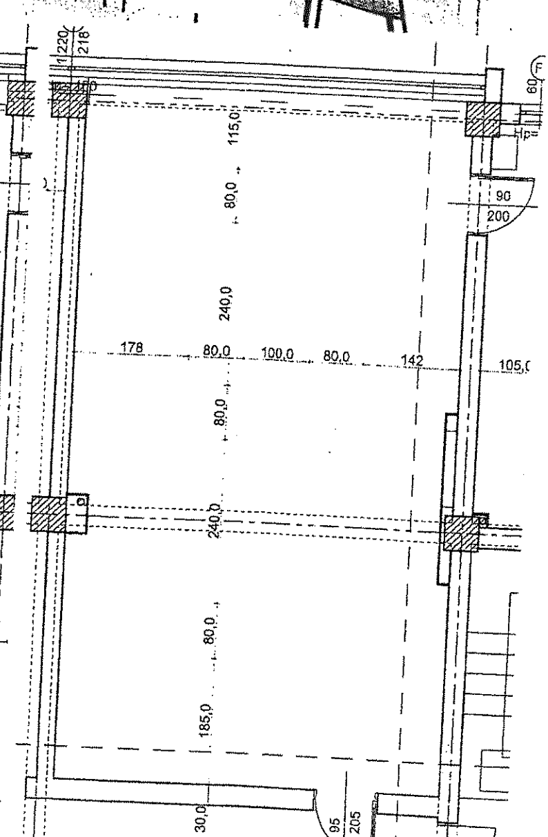
PLAN TAVAN - POZITIONARE CORPURI ILUMINAT
