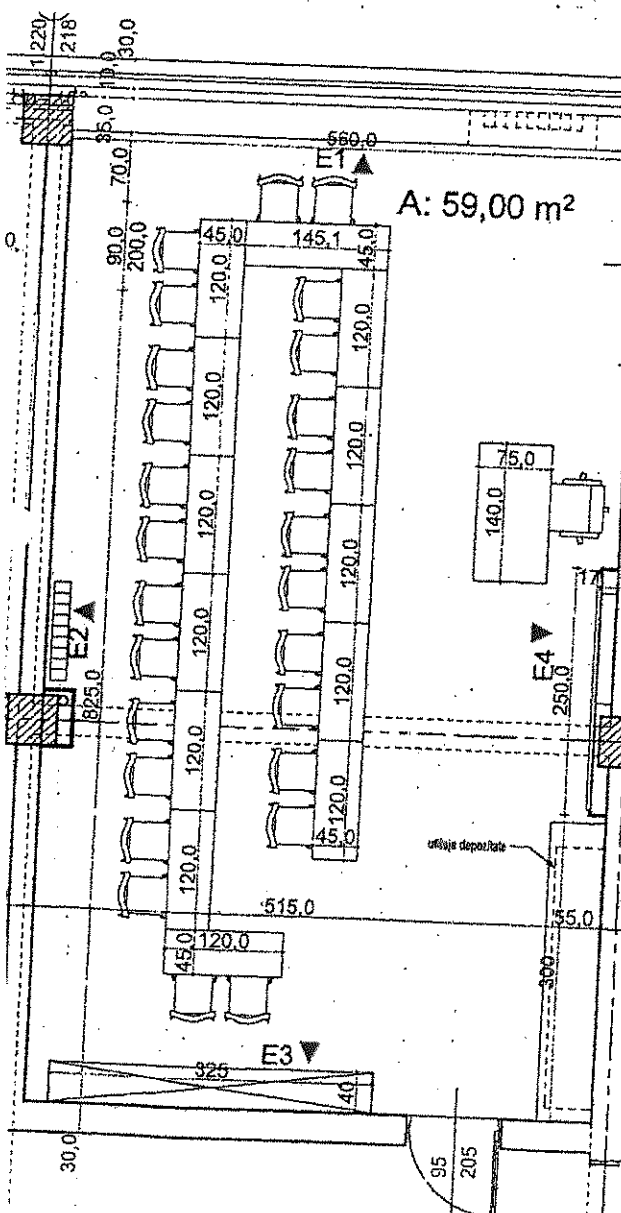
PLAN SALA DE CLASA
