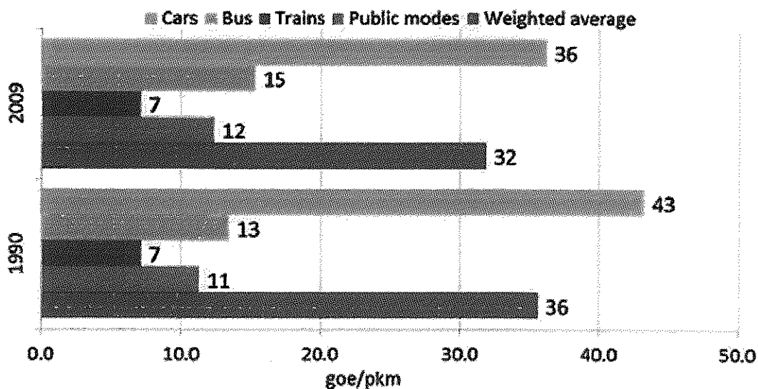
Figura 2 Comparație între consumul specific de energie funcție de modul de transport, în grame echivalent petrol pe persoană și km
