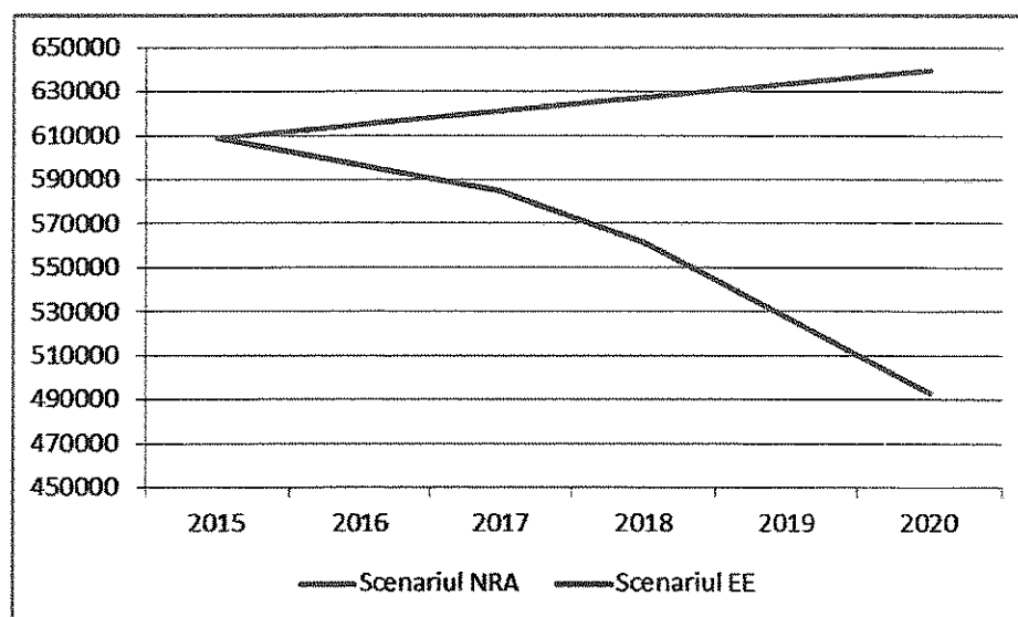
Figura 12 Evolutia consumului final de energie în cele doua scenarii analizate în perioada 2015 – 2020
