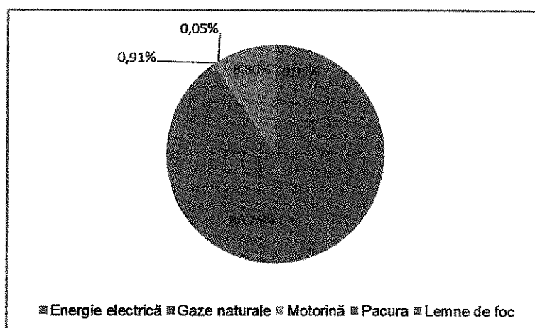
Figura 10 Structura consumului final de energie, anul 2015
