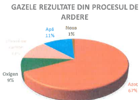
Figura 4.12. Compoziția gazelor rezultate din arderea motorinei.
