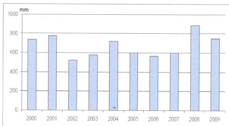
Variația precipitațiilor medii anuale (2000-2009)
